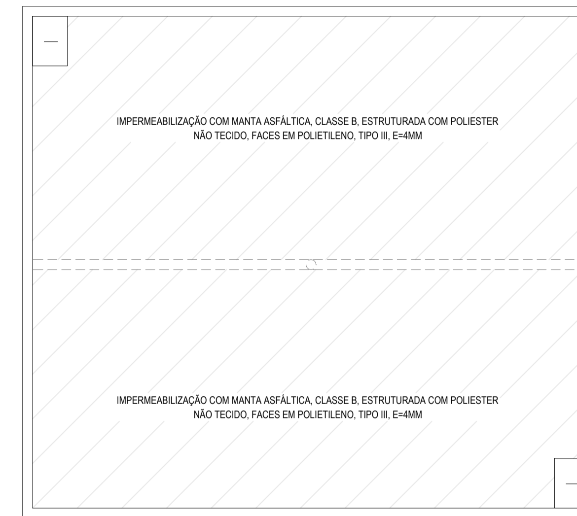
02 LAJE DE COBERTA ESC.: 1/75
