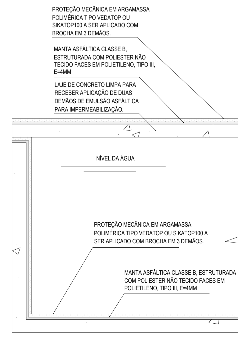
04 DETALHE DE IMPERMEABILIZAÇÃO DA COBERTA ESC.: 1/20
