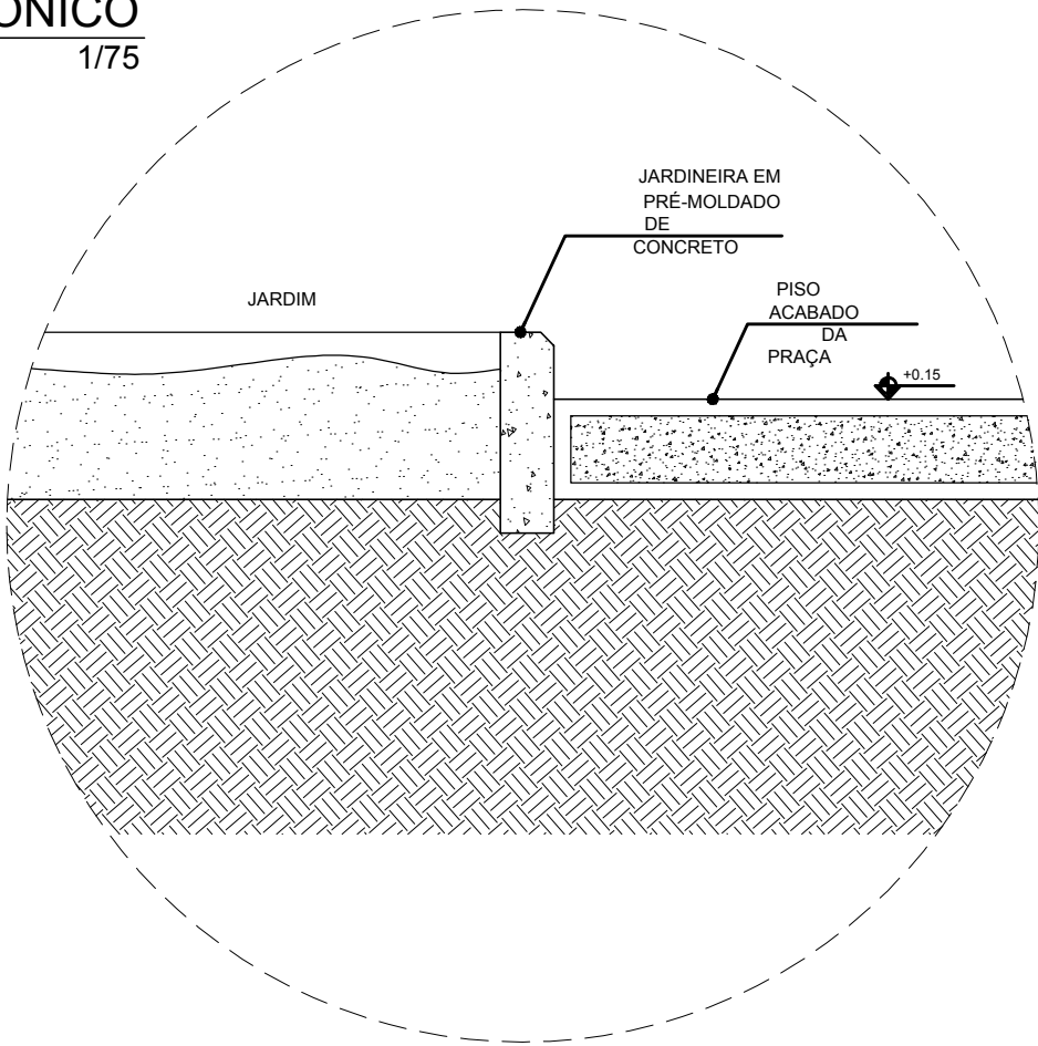
04 DET. JARDINEIRA PROJETO ARQUITETÔNICO ESCALA SEM ESCALA
