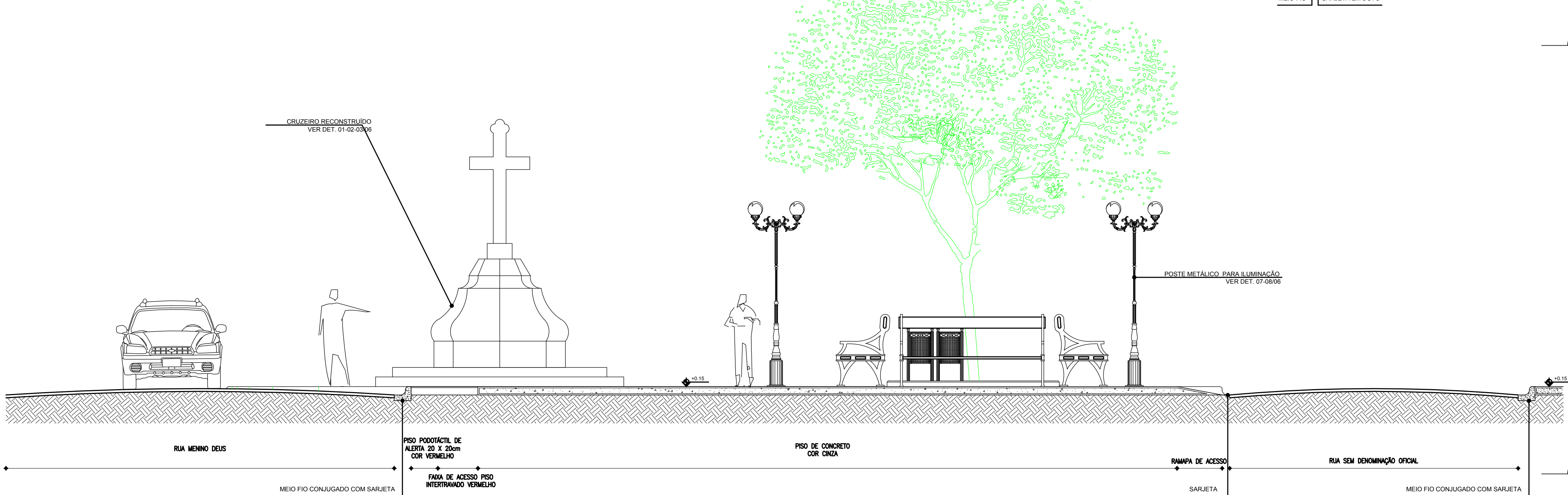
01 CORTE AA PROJETO ARQUITETÔNICO ESCALA 1/75
