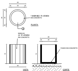
2 DETALHAMENTO LINEIRA ESCALA 1/20
