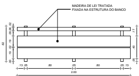
1 DETALHAMENTO BANCO ESCALA 1/20
