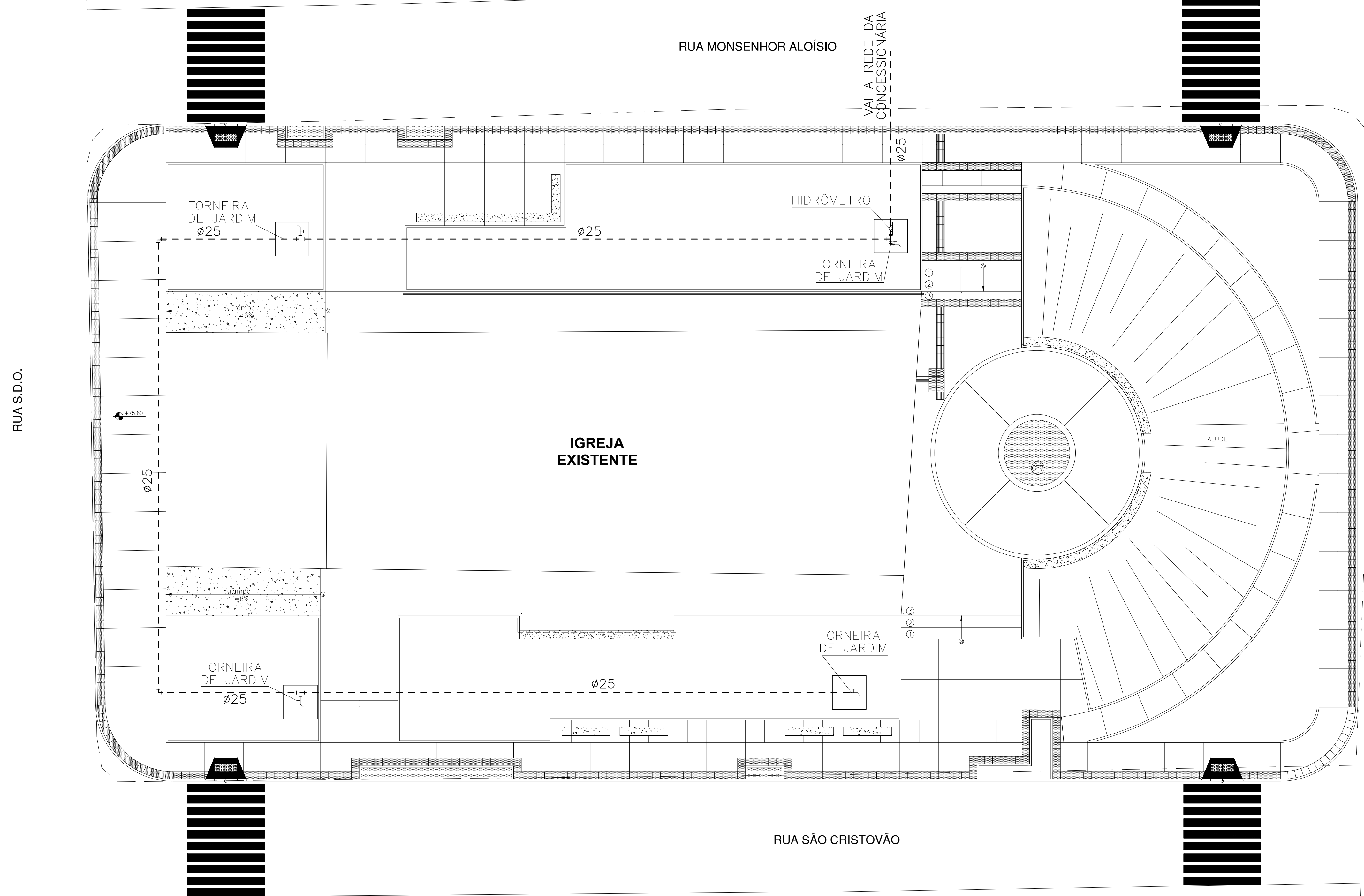
PLANTA BAIXA ESCALA 1/125
