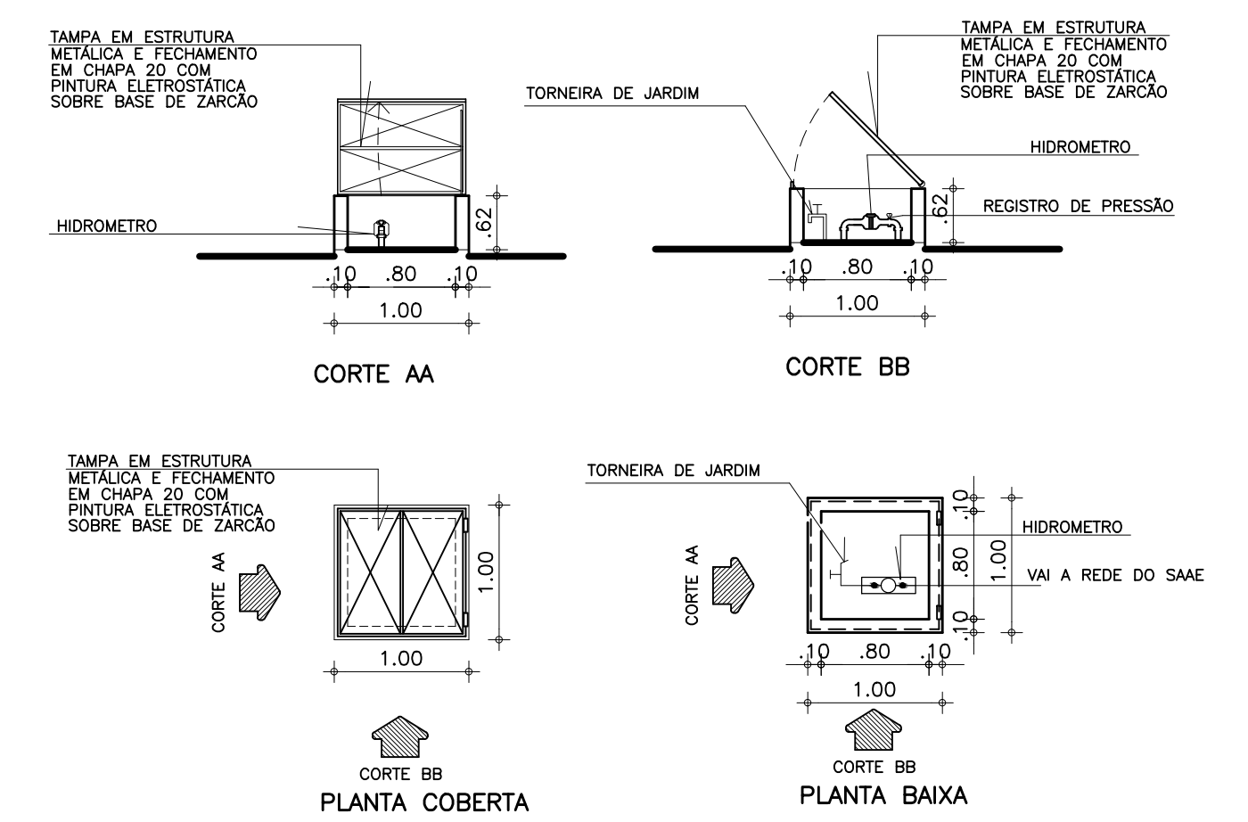
DETALHE CAIXA HIDROMETRO PARA PRAÇA SEM ESCALA
