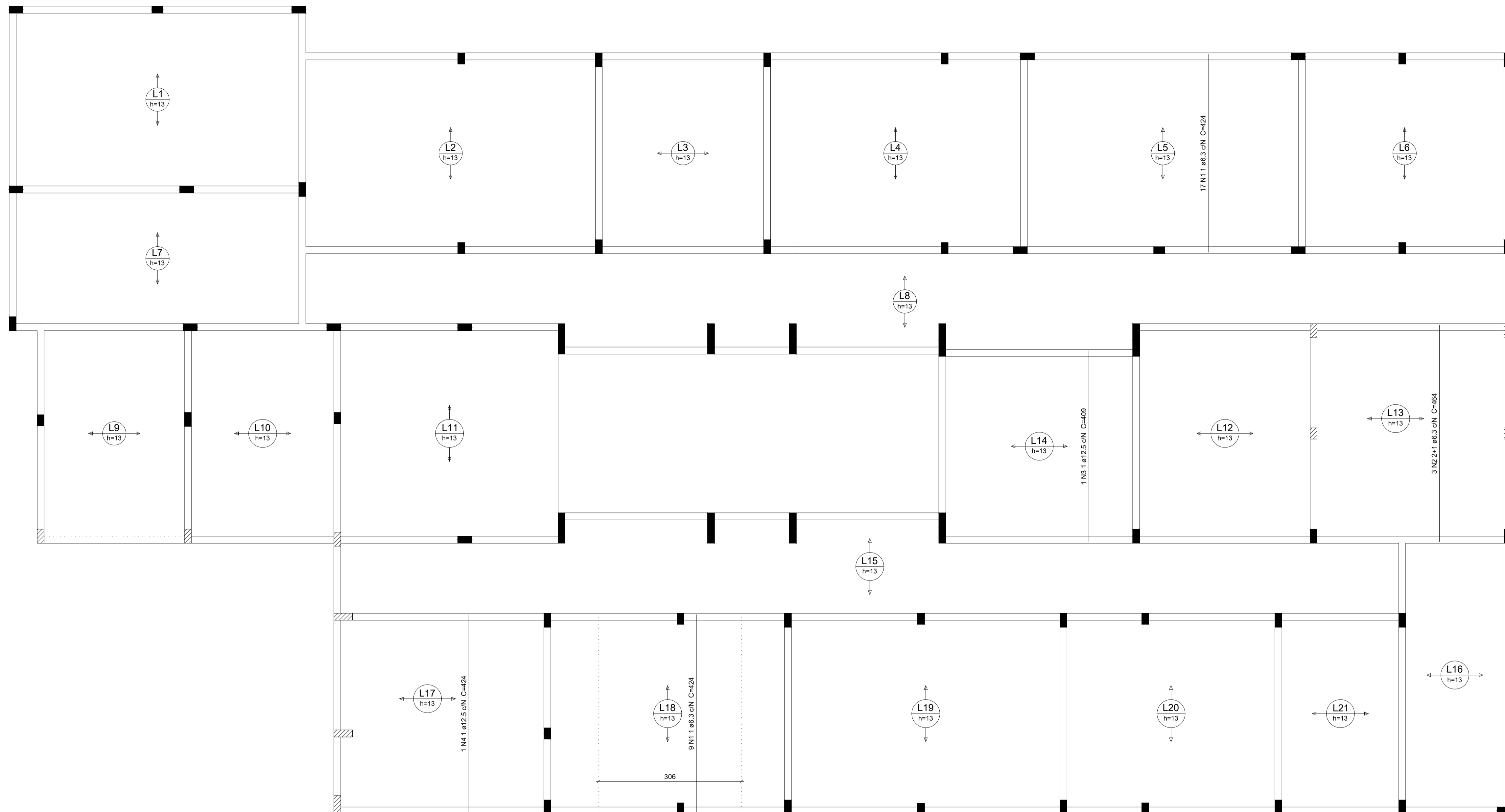
Armação positiva das lajes do pavimento TIPO (Eixo Y)
