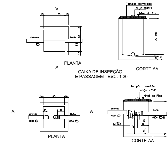
CAIXA DE GORDURA - ESC. 1:20 - CAIXA DE GORDURA dupla (CGD), PRISMÁTICA [NBR 8162:1999 - 5.1.5.1.3a]
