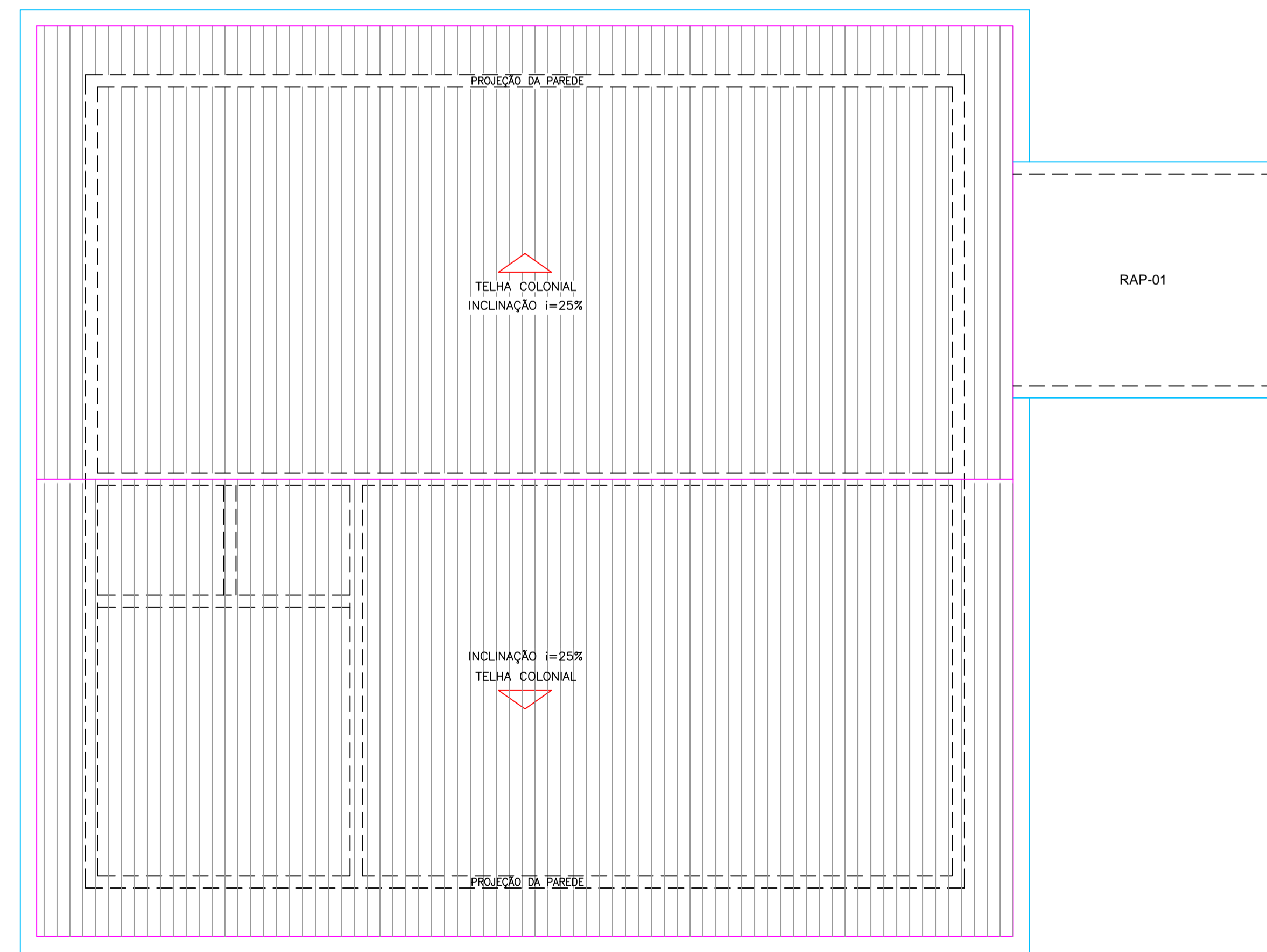
02 PLANTA DE COBERTA ESCALA: 1/50
