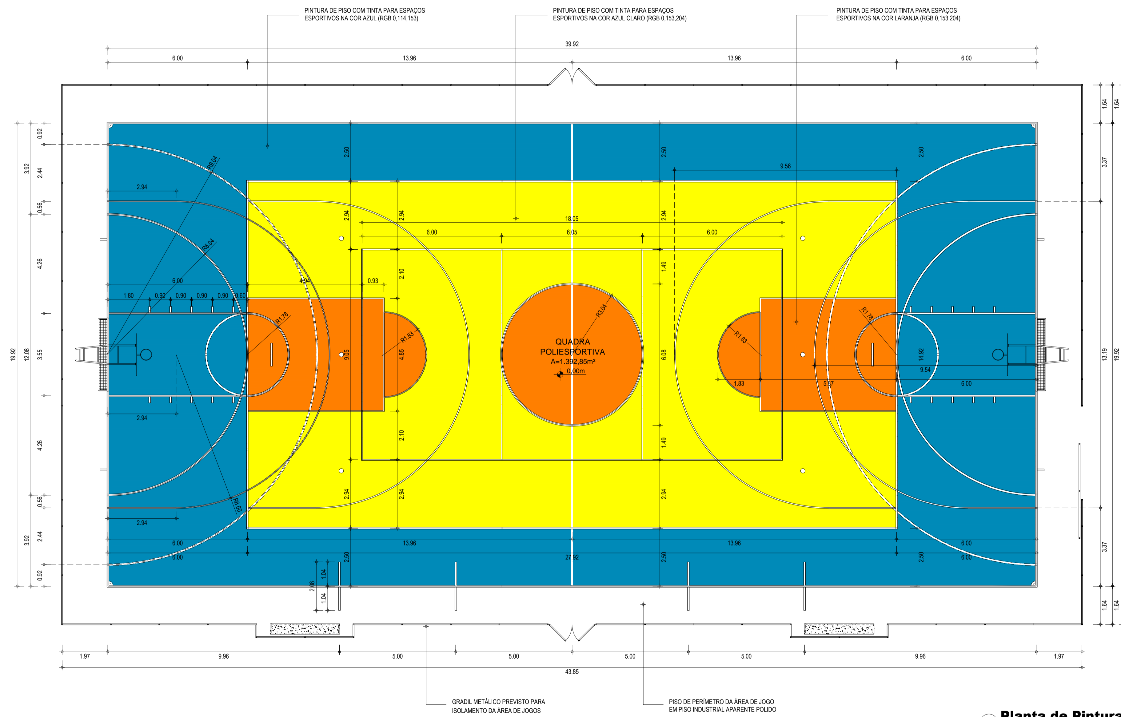
18 Planta de Pintura - Quadra ESCALA 1/100
