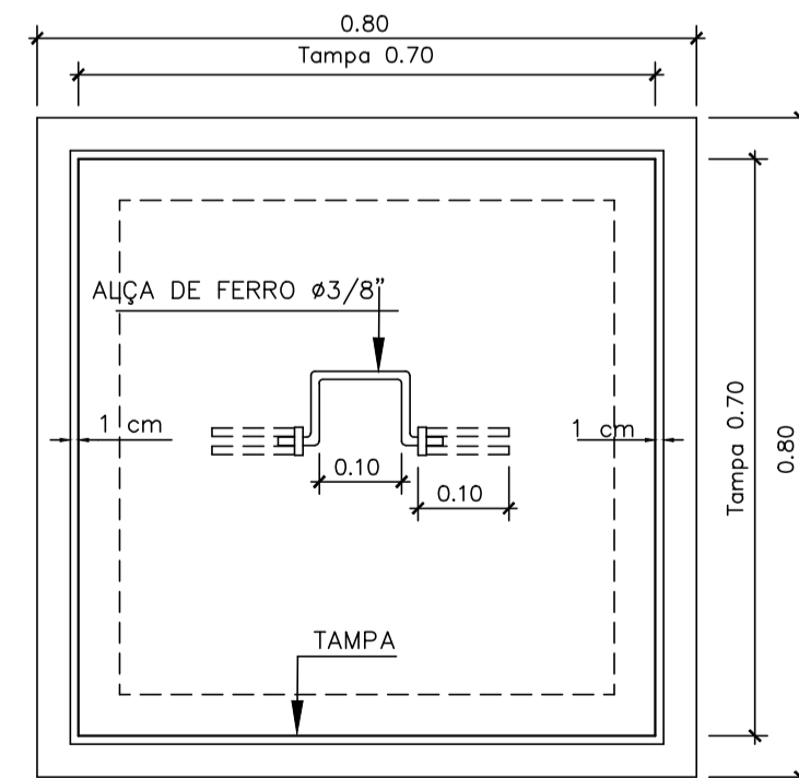
VISTA SUPERIOR.
