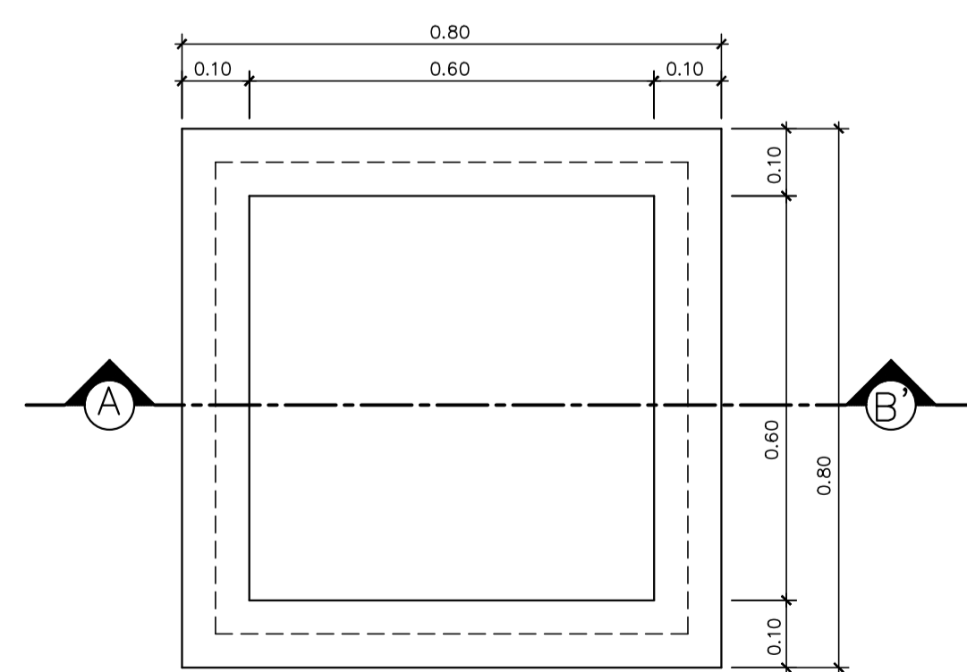
PLANTA BAIXA
