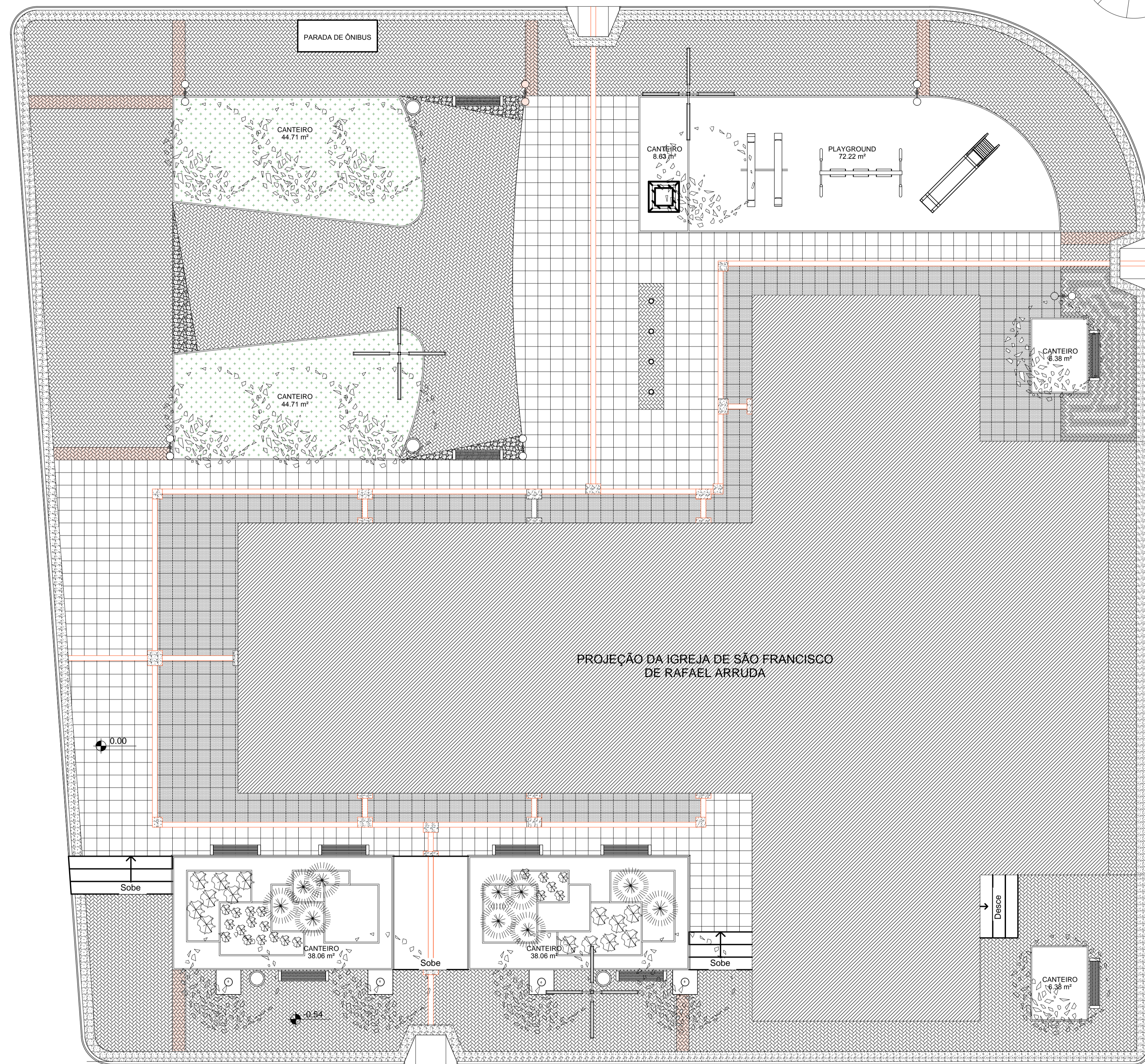
02 PLANTA GERAL ESCALA 1/100
