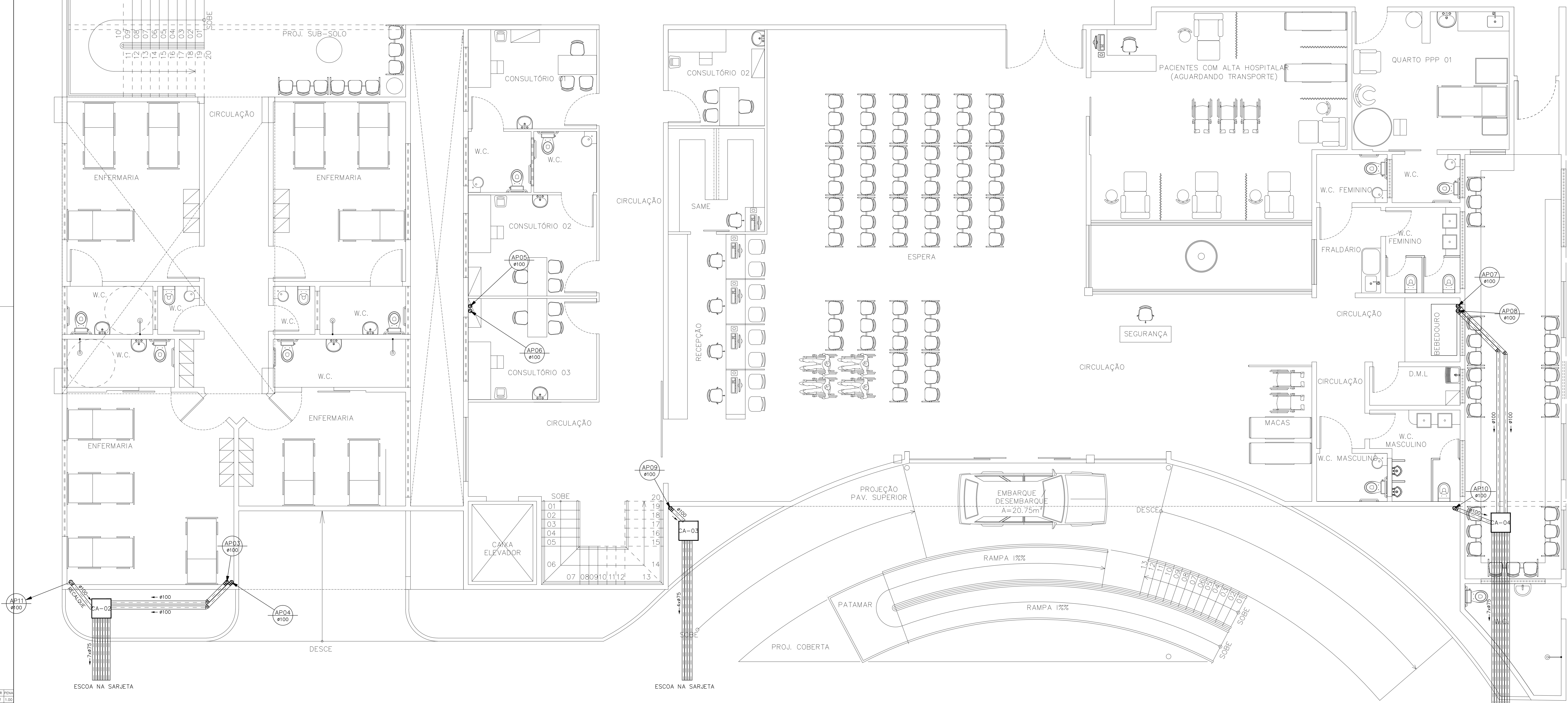
PLANTA BAIXA TÉRREO ESCALA 1/50
