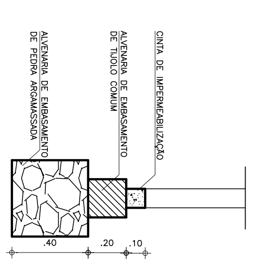
7 DETALHE DA FUNDAÇÃO ESCALA: 1:20
