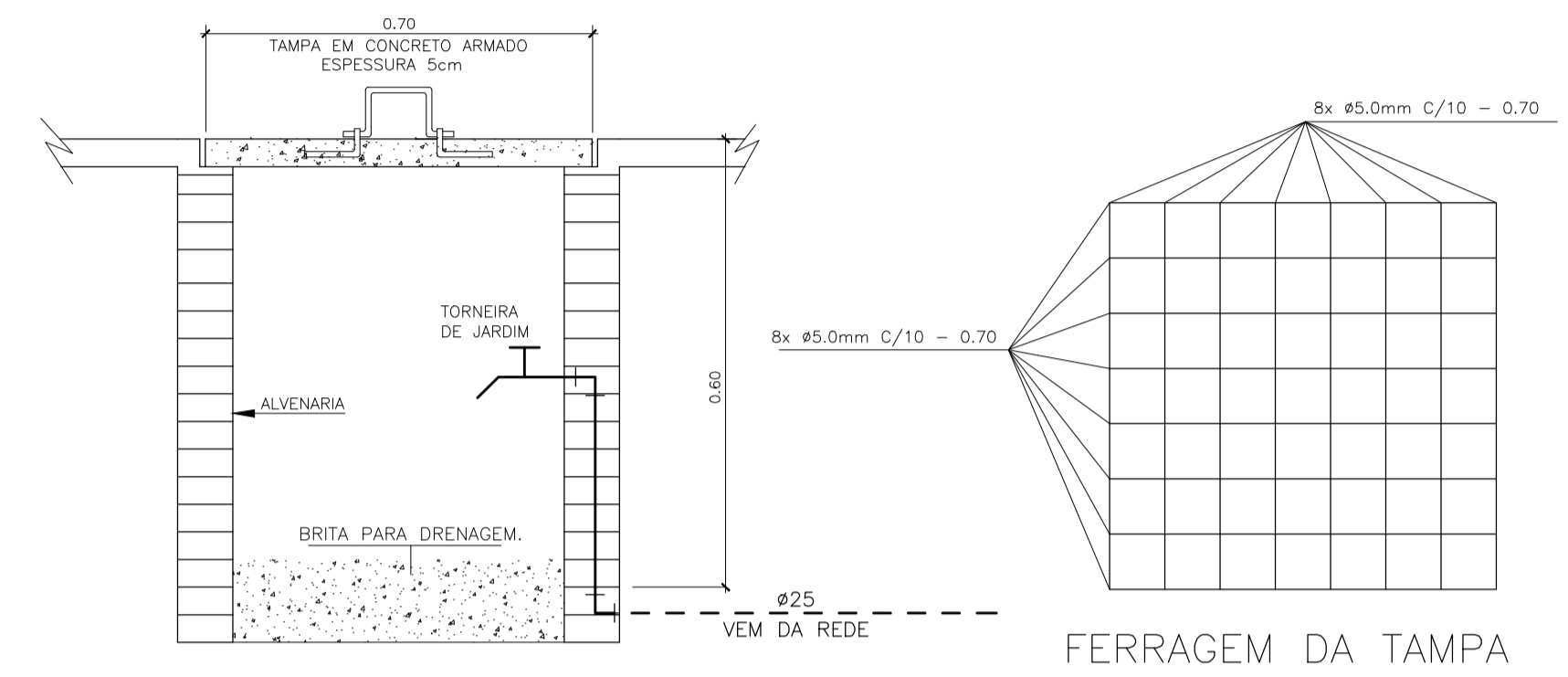
DETALHE EXECUTIVO DA CAIXA COM TORNEIRA DE JARDIM CAIXA DE PASSAGEM 60x60x60cm - TAMPA DE CONCRETO
