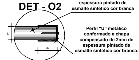
DETALHE PAINEL DO MÓDULO - 01 Escala: 1/1
