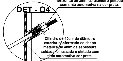
DETALHE DE FIXAÇÃO DO TENSOR DO MÓDULO - 01 Escala: 1/1
