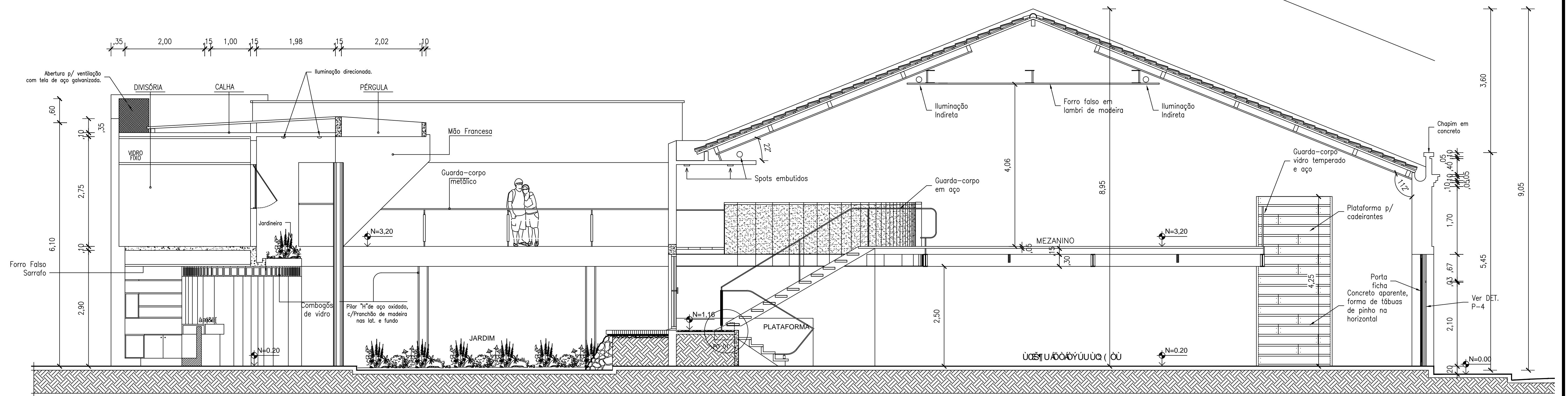
03 CORTE AA ESC. -- 1/50
