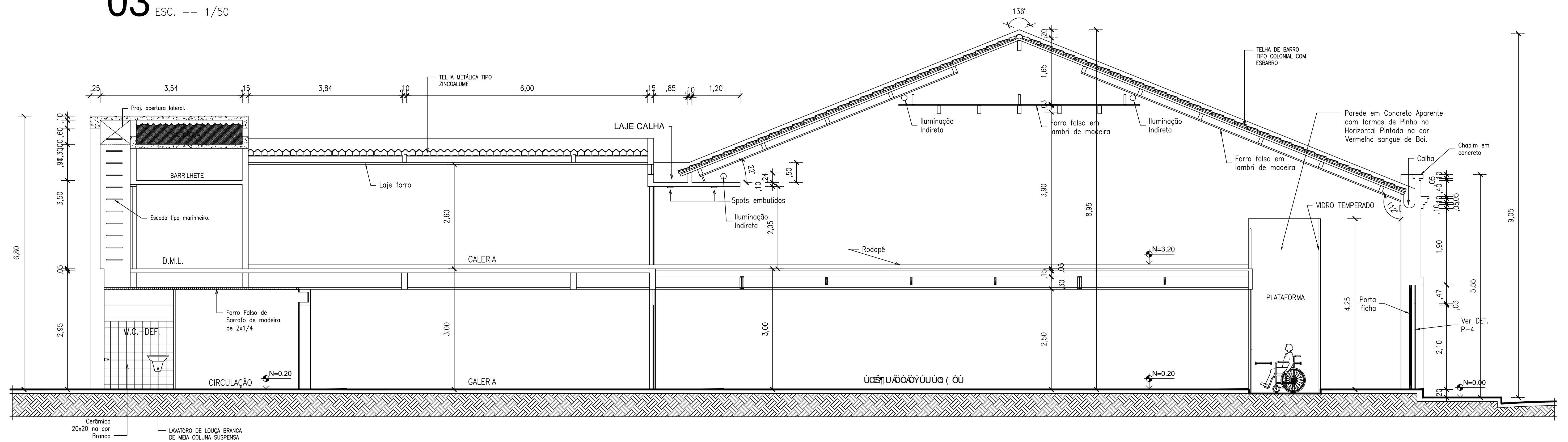
04 CORTE BB ESC. -- 1/50
