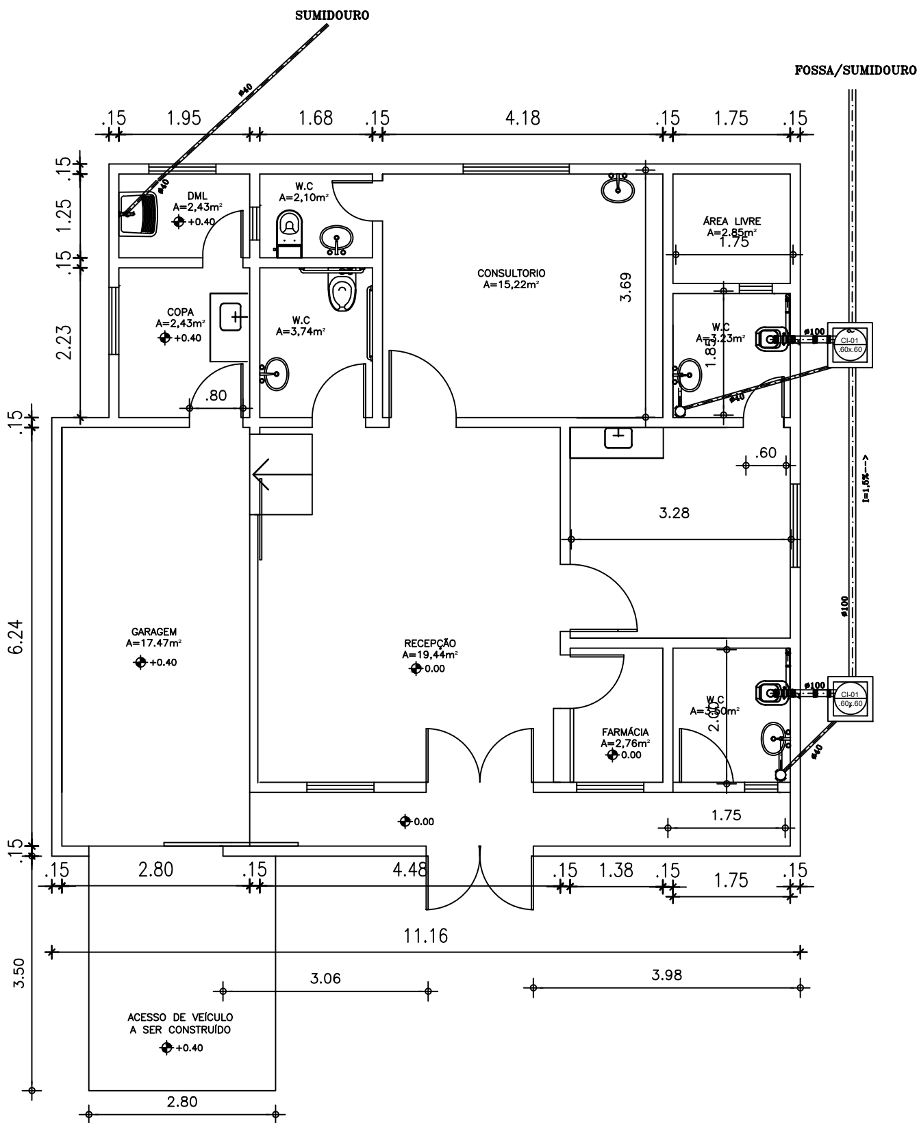
03 HIDROSSANITÁRIO ESCALA - 1: 100
