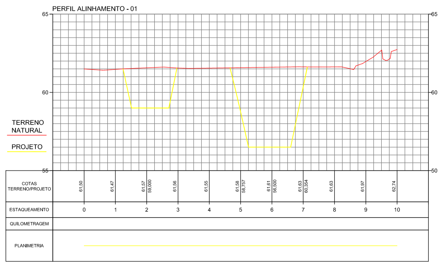
01 PERFIL LONGITUDINAL ESCALA — 1 : H: 1/1000 — V: 1/100
