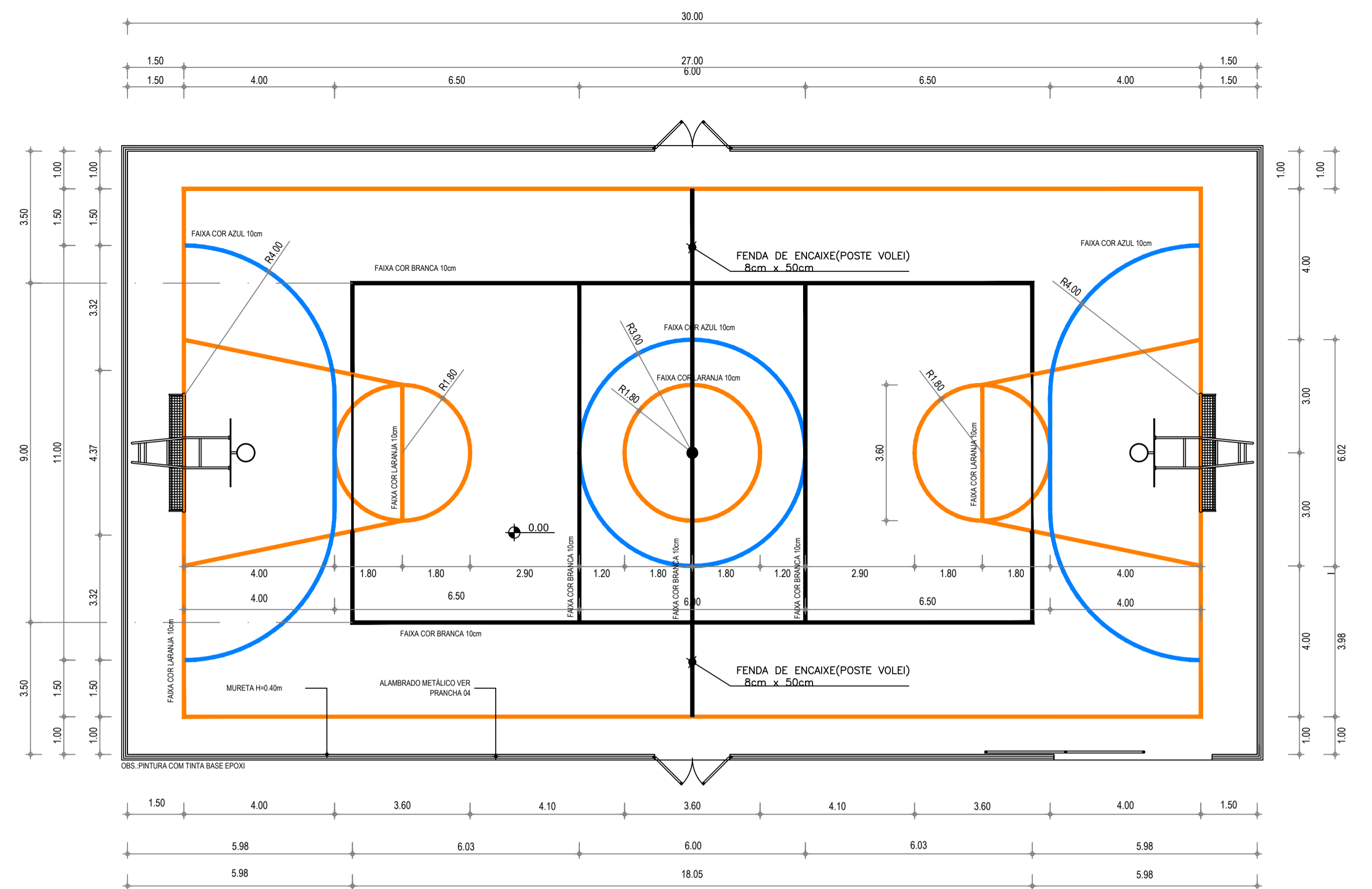
3 DEMARCAÇÃO E CORES QUADRA ESCALA 1/100
