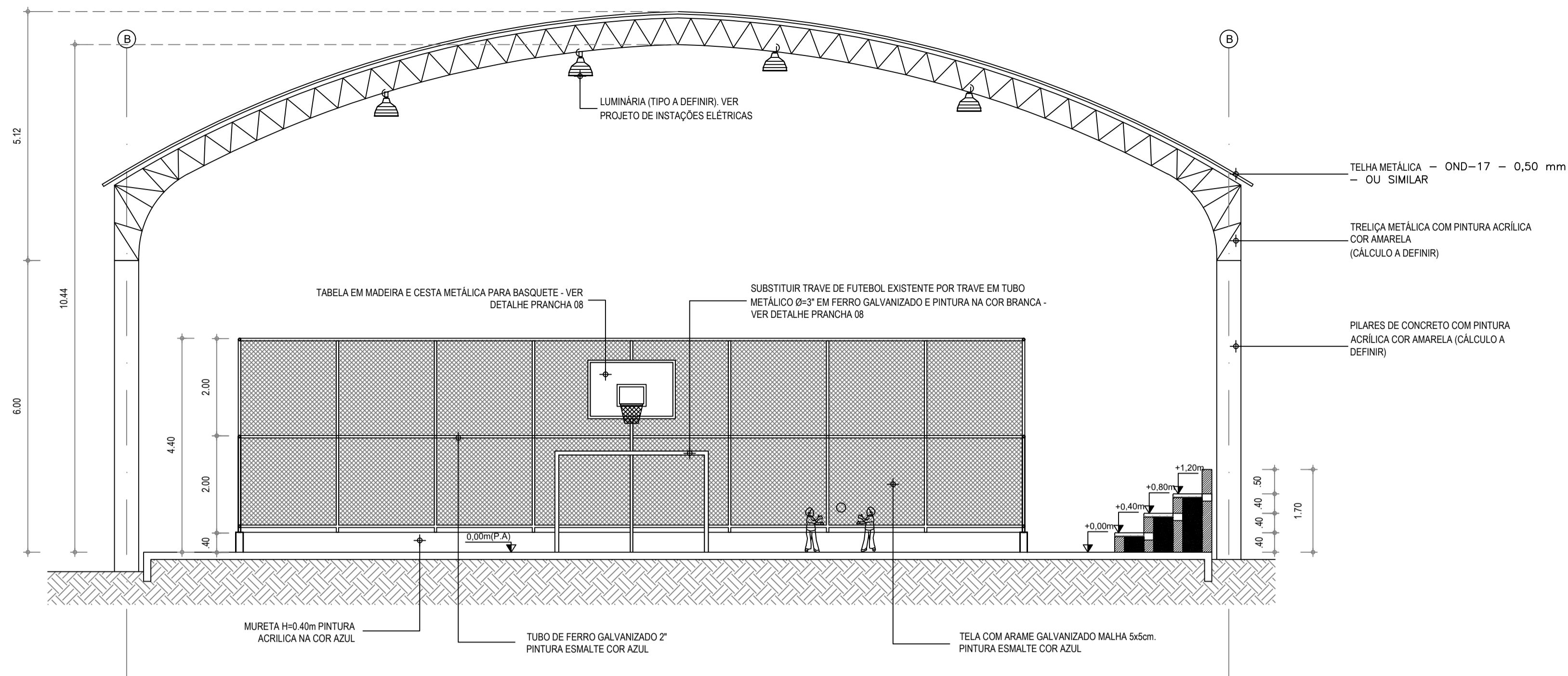
1 CORTE AA QUADRA ESCALA 1/75
