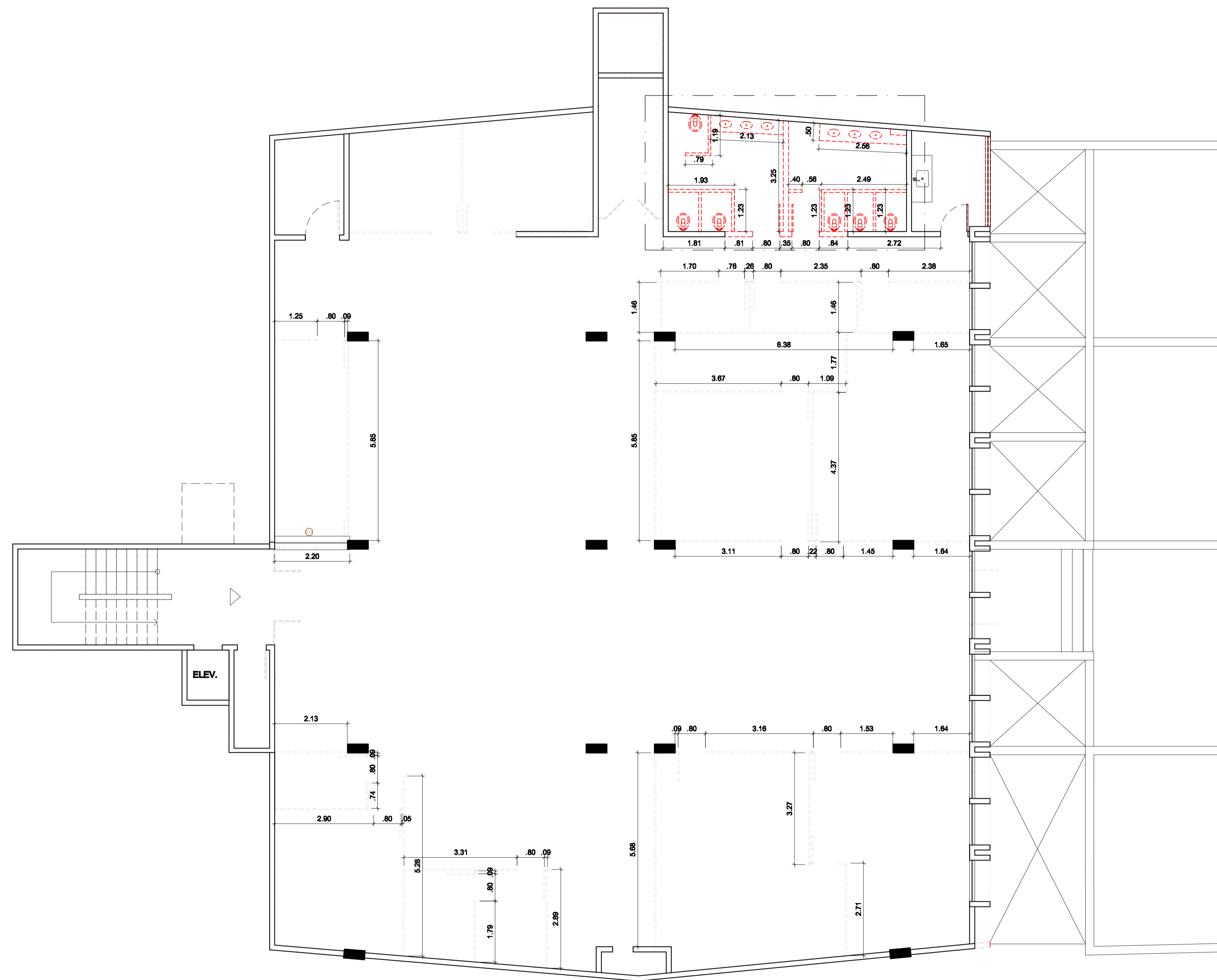
3 PLANTA DE DEMOLIÇÃO 2º ANDAR ESCALA 1/75
