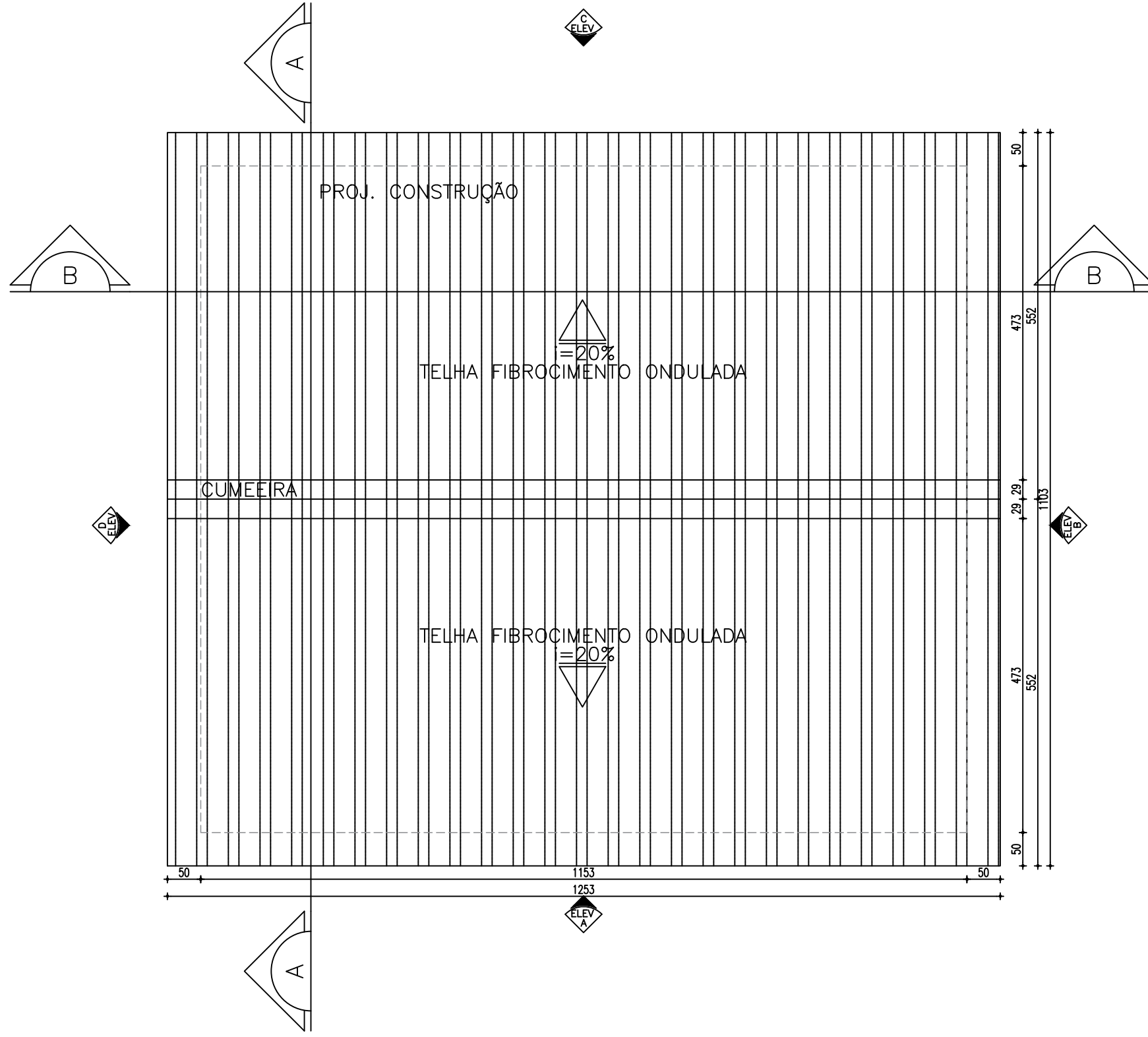
01 PLANTA BAIXA - COBERTA
