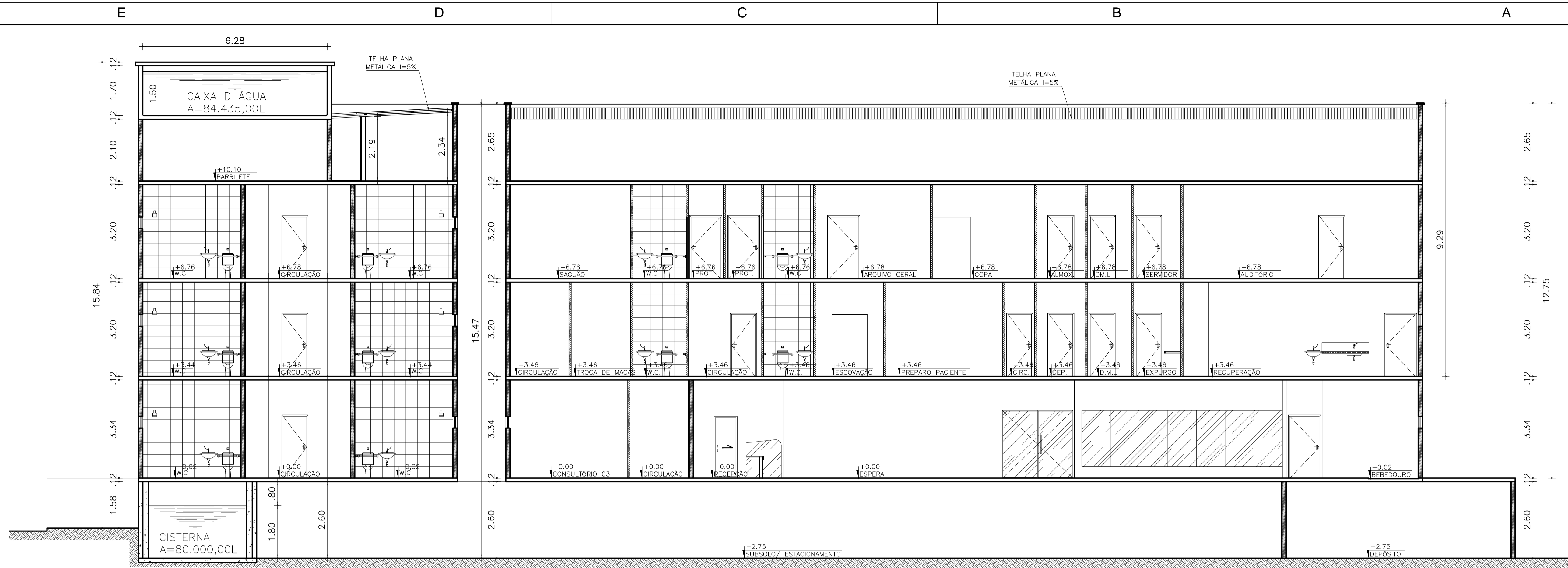
01 CORTE BB
