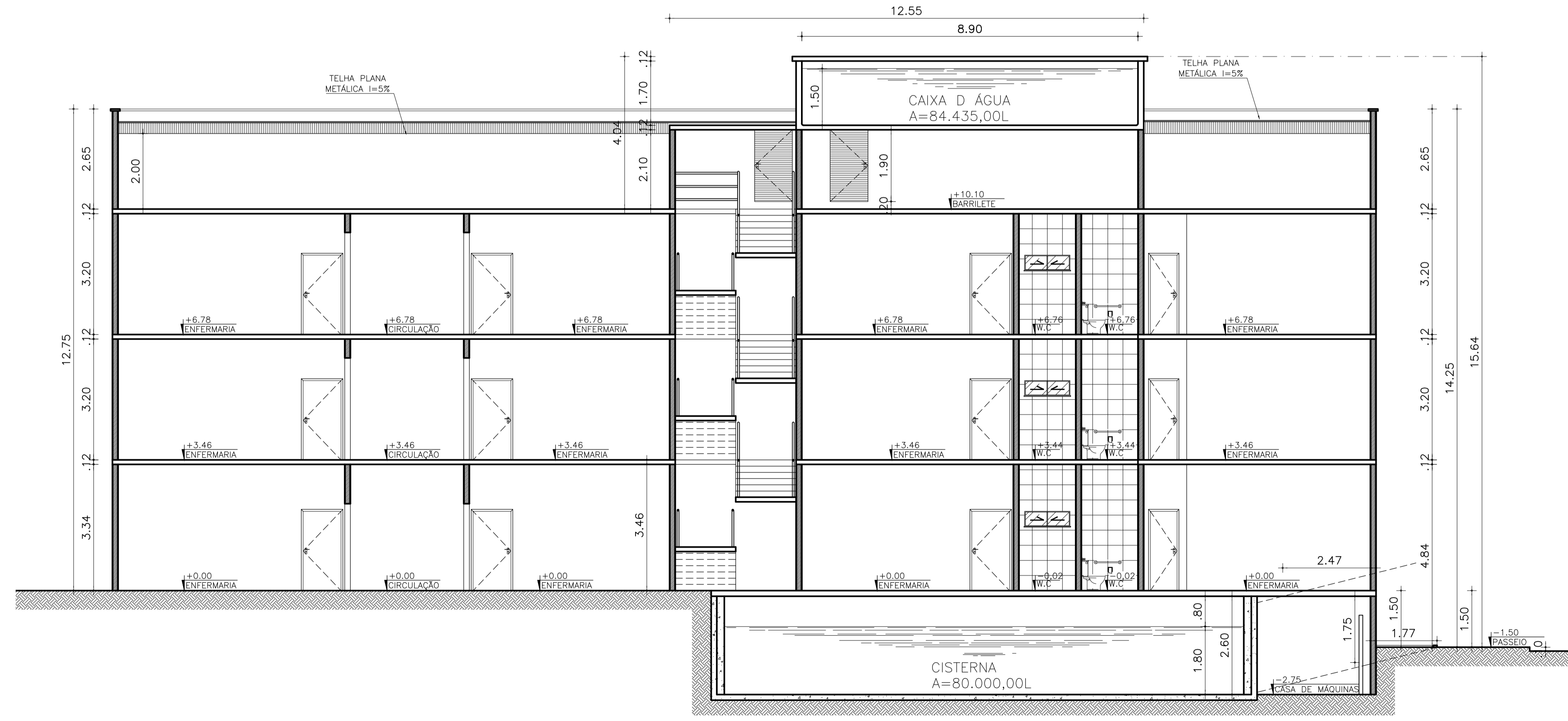
02 CORTE AA
