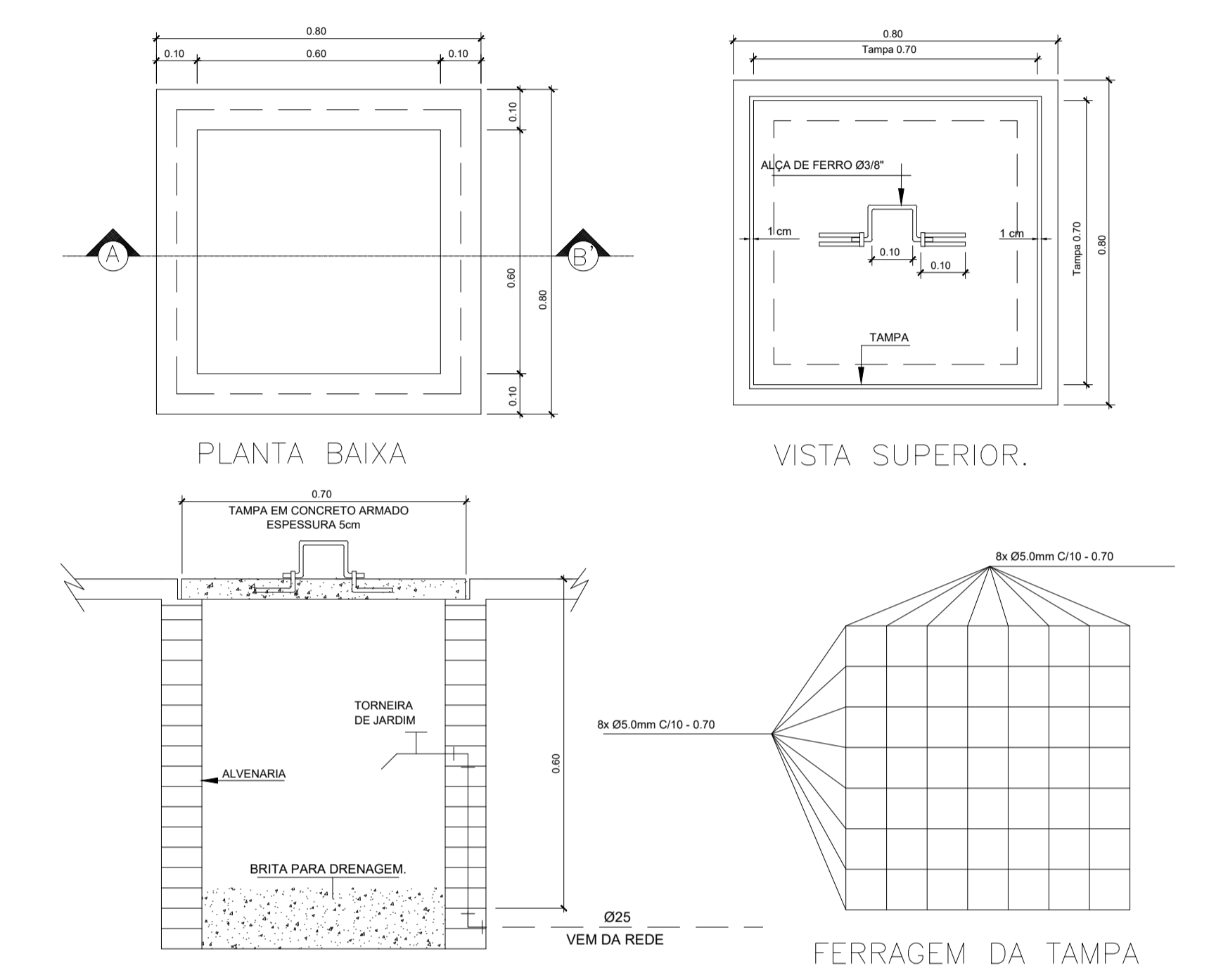
DETALHE EXECUTIVO DA CAIXA COM TORNEIRA DE JARDIM CAIXA DE PASSAGEM 60x60x60cm - TAMPA DE CONCRETO
