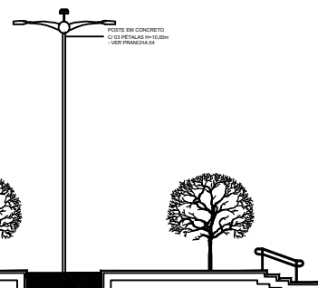
2 CORTE BB ESCALA 1/50
