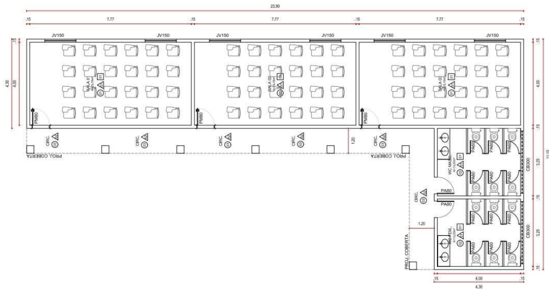
Figura. 04 Planta Baixa - Sobral, CE. Fonte: SEINFRA (editado pelo autor)
