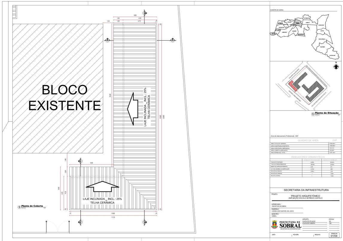
Figura. 03 Implantação - Sobral, CE. Fonte: SEINFRA (editado pelo autor)
