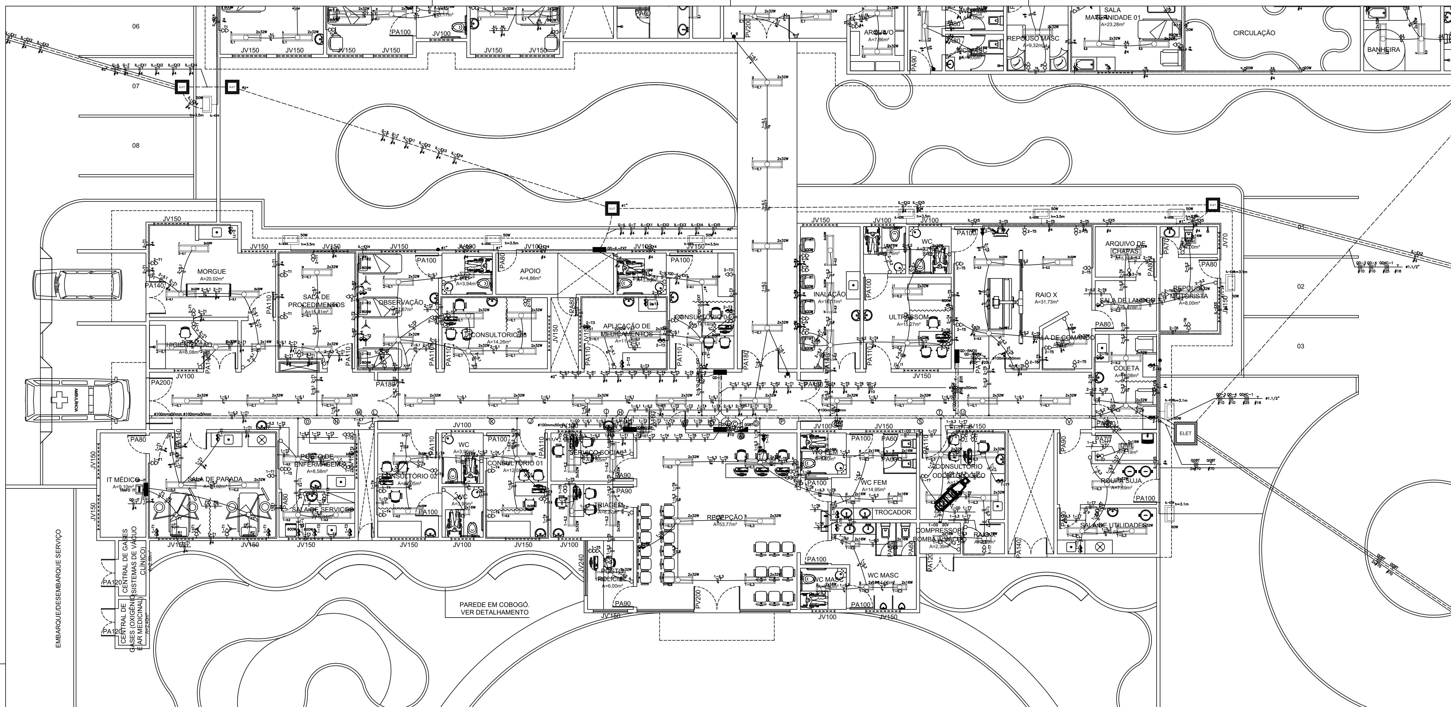
1 PLANTA BAIXA - BLOCO 1 ESCALA 1/100
