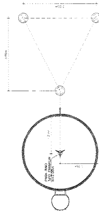
PLANTA BAIXA ATERROAMENTO PARA-RAIO
