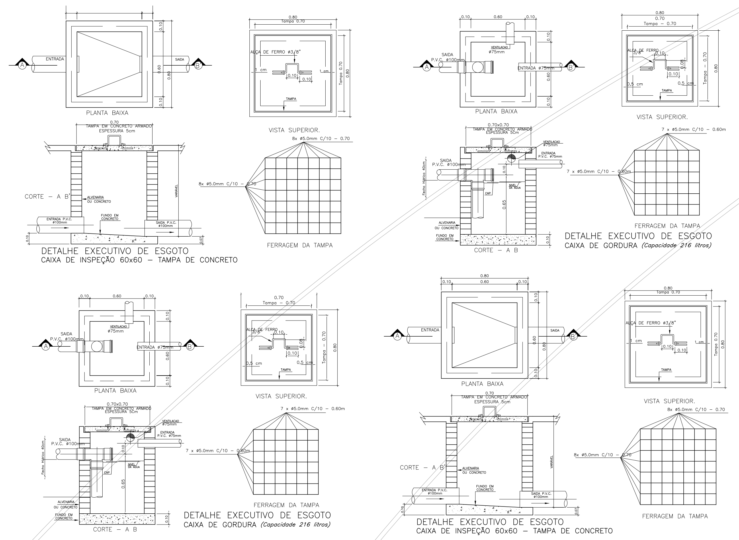
02 DETALHES CAIXAS 1/20
