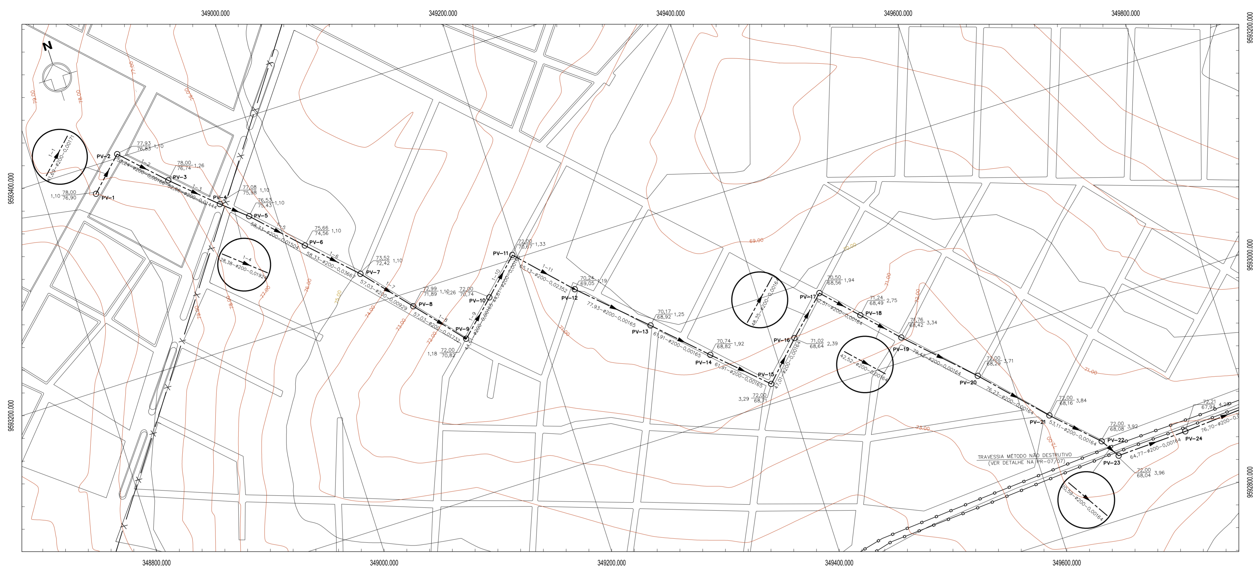
PLANTA BAIXA - COLETOR EMISSÁRIO ESCALA: 1/2000
