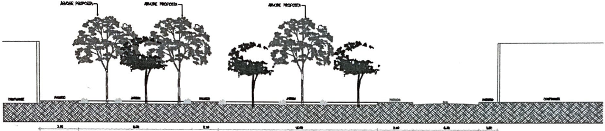
02 CORTE BB 1/100
