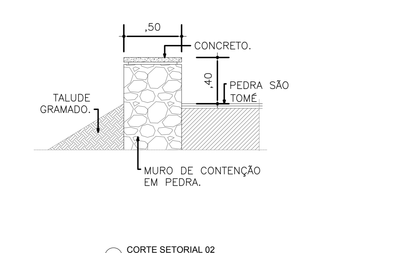
07 CORTE SETORIAL 02 1/75
