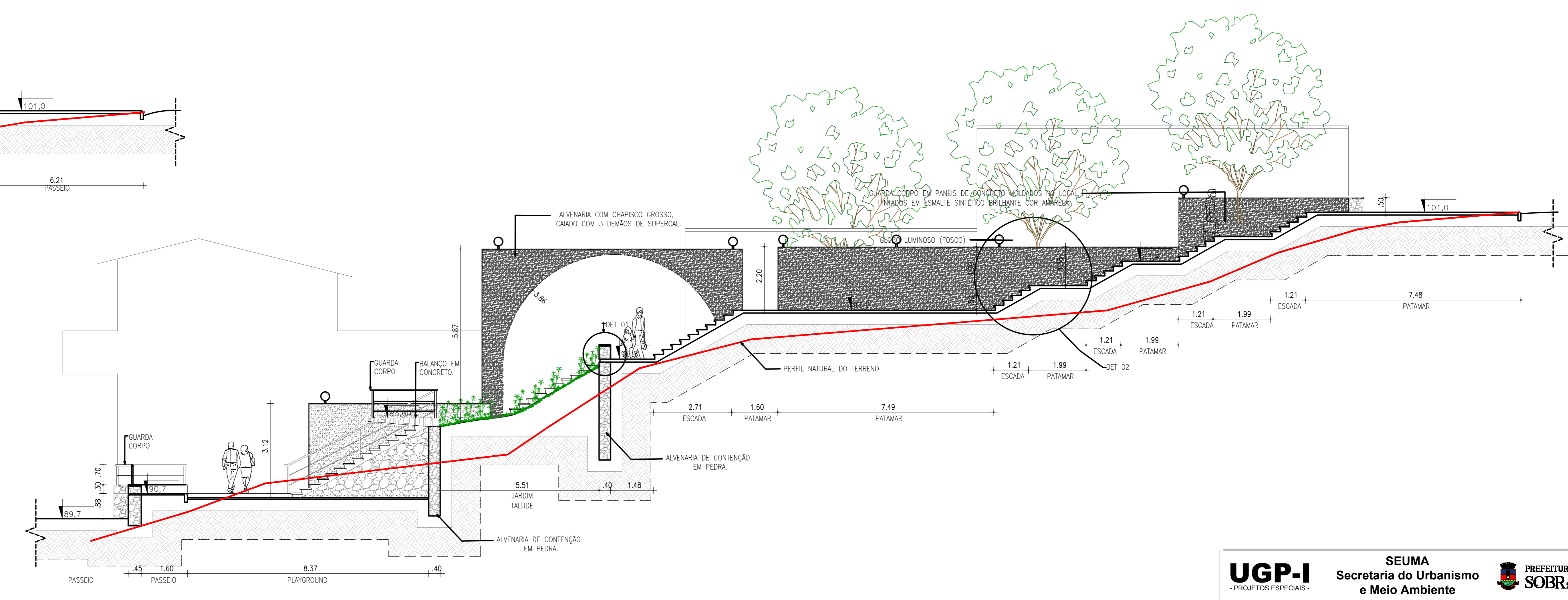
04 CORTE BB 1/75
