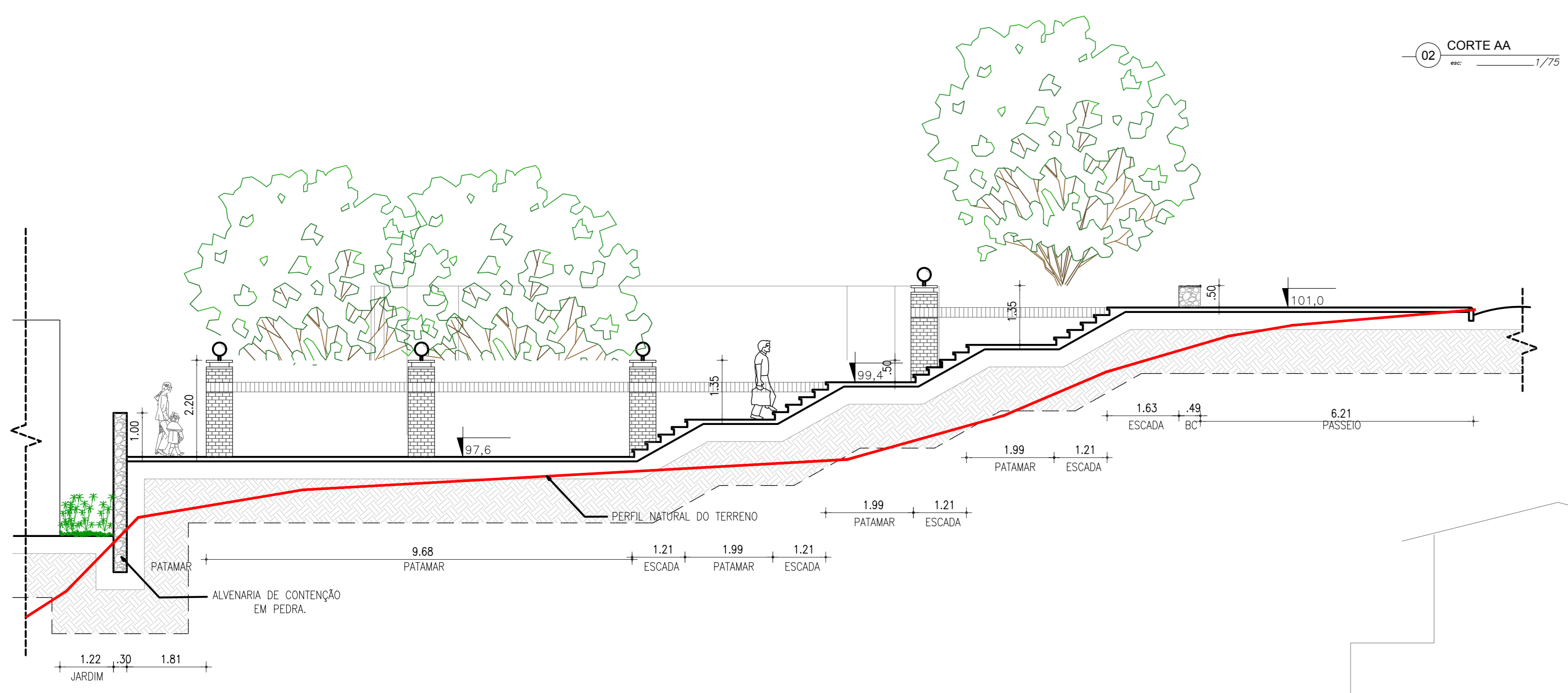
03 CORTE CC 1/75
