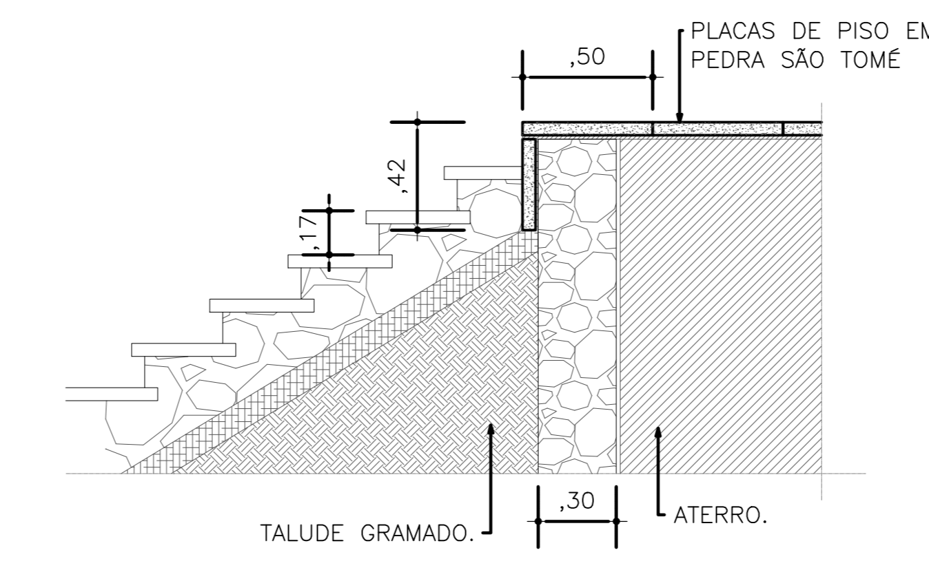
06 CORTE SETORIAL 01 1/75
