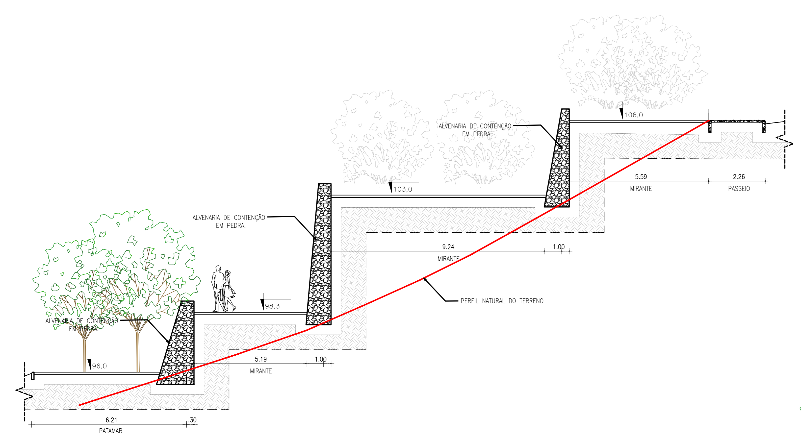
01 CORTE SETORIAL - 03 1/75
