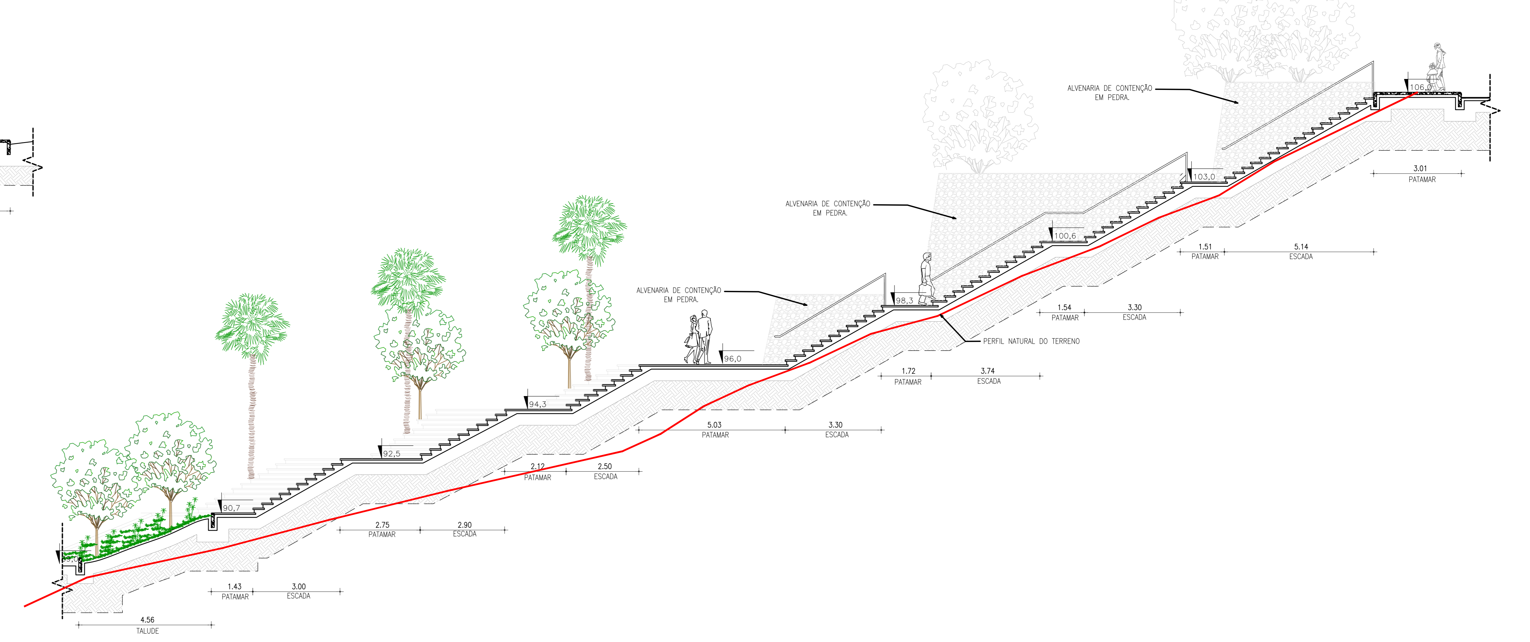
02 CORTE AA 1/75
