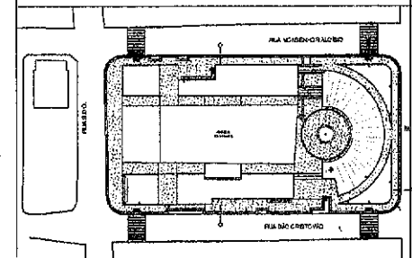
01 PLANTA BAIXA SITUAÇÃO
