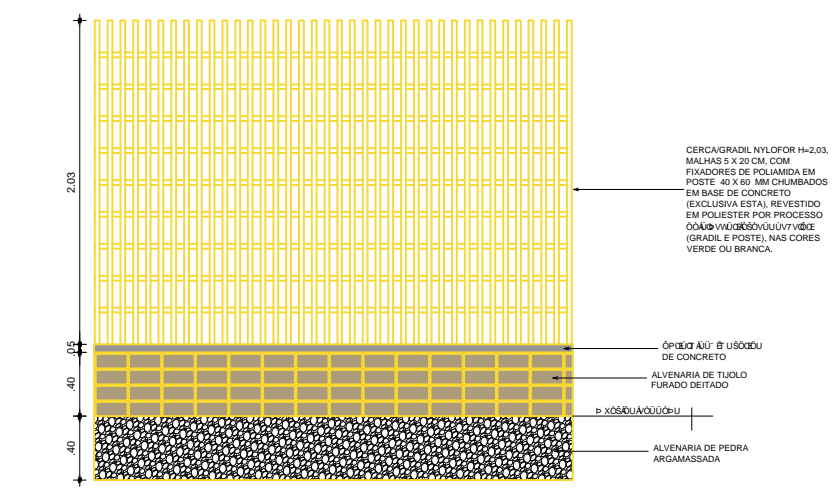
2 DETALHAMENTO DE GRADIL - CORTE LONGITUDINAL SEM ESCALA
