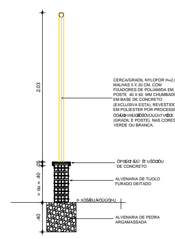
3 DETALHAMENTO DE GRADIL - CORTE TRANSVERSAL SEM ESCALA
