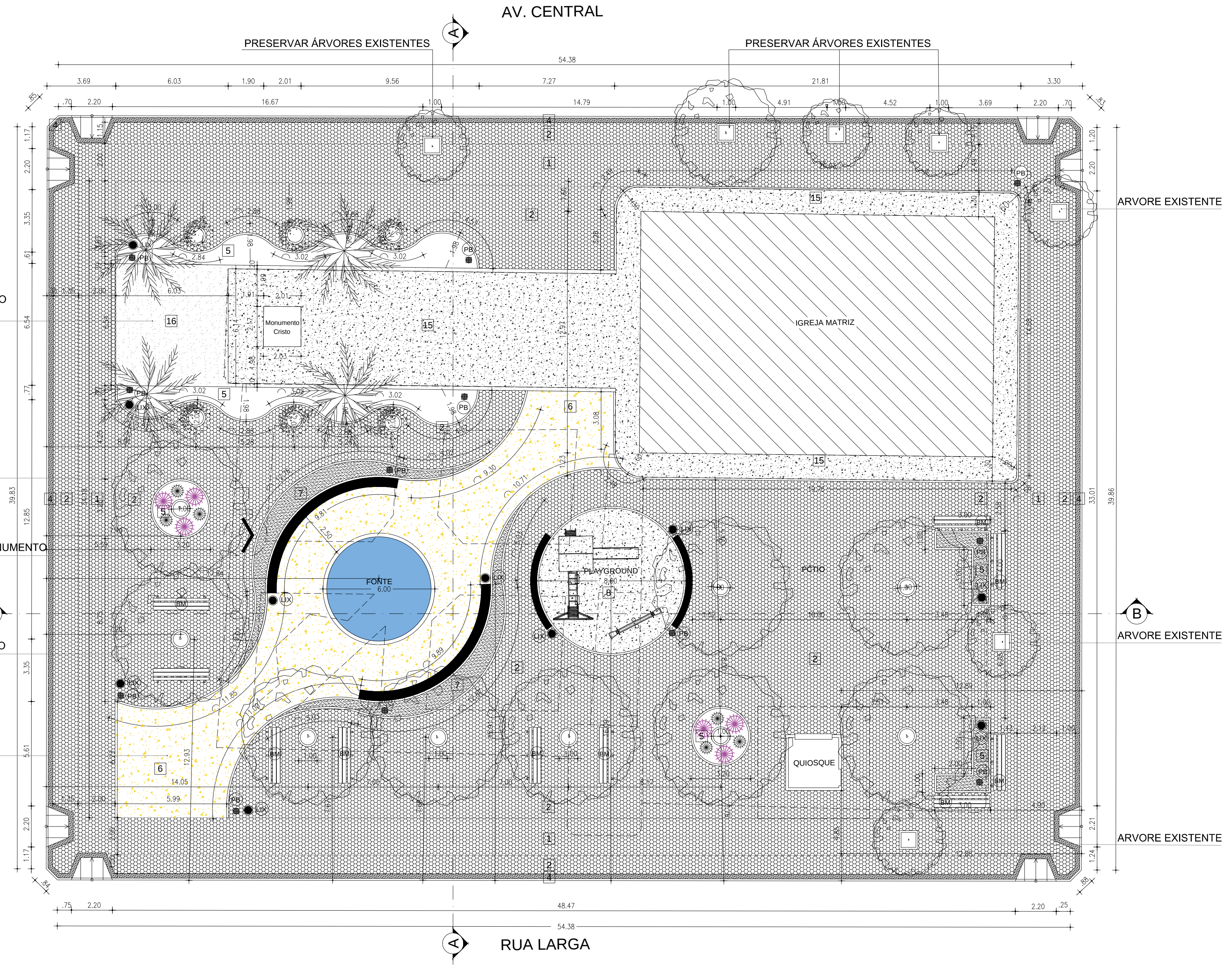
02 PLANTA GERAL esc 1/150
