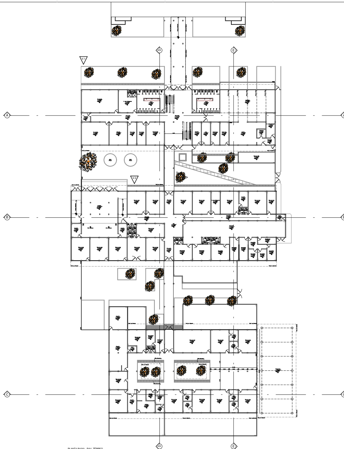
1 PLANTA BAIXA - PAV. TERREO ESCOLA DO CAIC ESCALA 1/200
