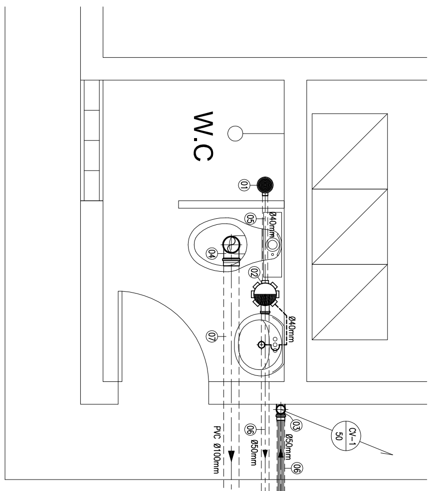
WC - INSTALAÇÃO SANITARIA ESCALA 1:25
