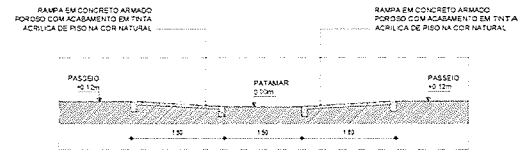
4 DETALHAMENTO RAMPA ESCALA 1/50
