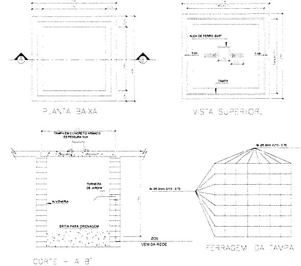
DETALHE EXECUTIVO DA CAXA COM TORNEIRA DE LARDAIV CAXA DE PASSAGEM 60x60x60cm - TAVPA DE CONCRETO
