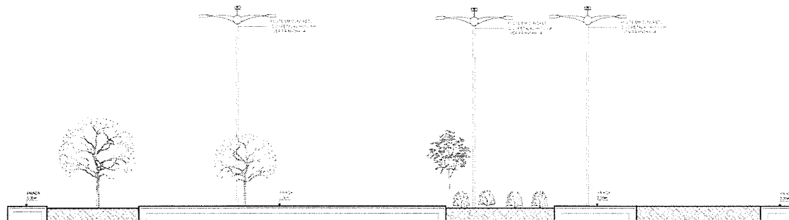
1 CORTE AA Escala 1:50
