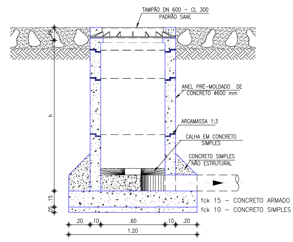
POÇO DE VISITA DE CABECEIRA - Ø 600 mm
