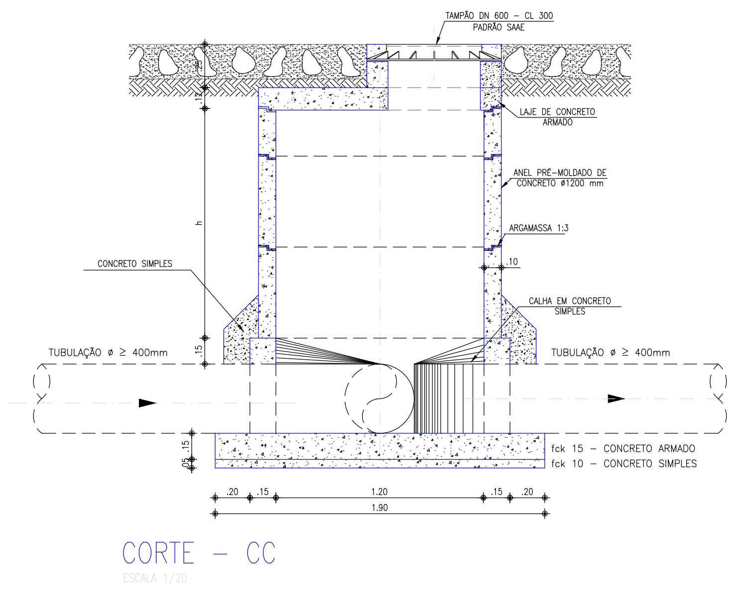
POÇO DE VISITA Ø 1200 mm
