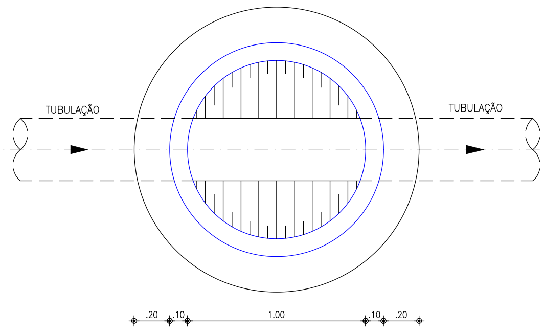
POÇO DE VISITA Ø 1000 mm
