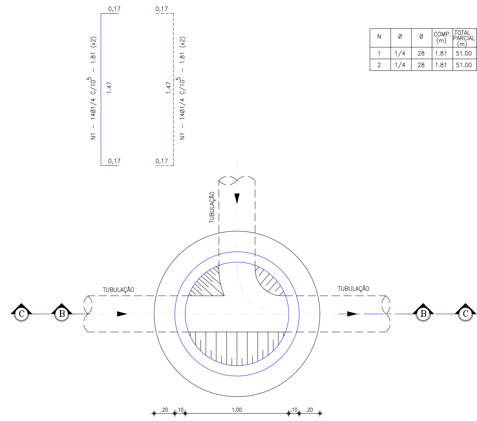
POÇO DE VISITA Ø 1200 mm
