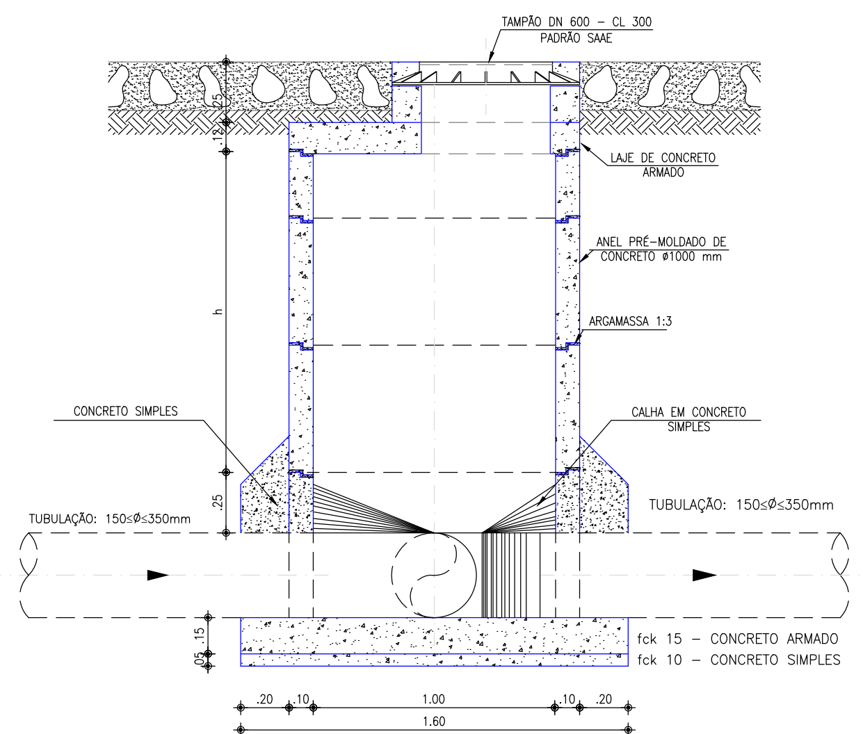
POÇO DE VISITA Ø 1000 mm
