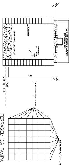
DETALHE EXECUTIVO DA CAIXA COM TORNEIRA DE JARDIM CAIXA DE PASSAGEM 60x60x60cm - TAMPA DE CONCRETO
