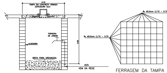
CORTE - A B'
