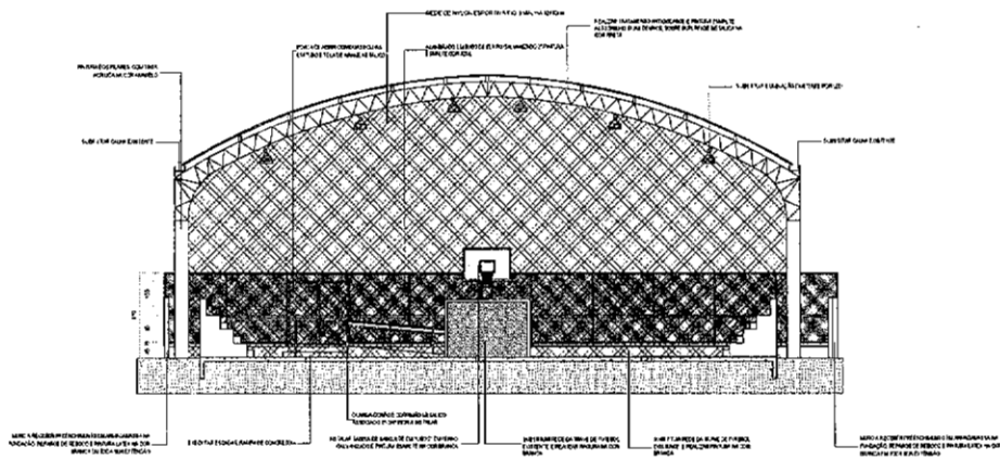
2 Corte BB - Quadra ESCALA 1/50
