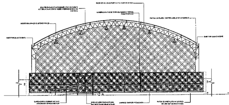
3 Vista 01 - Quadra ESCALA 1/50
