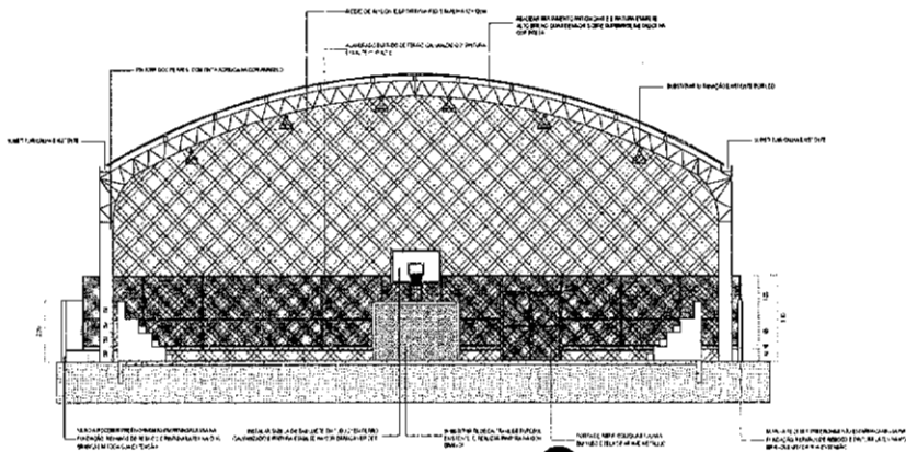
3 Corte CC - Quadra ESCALA 1/50
