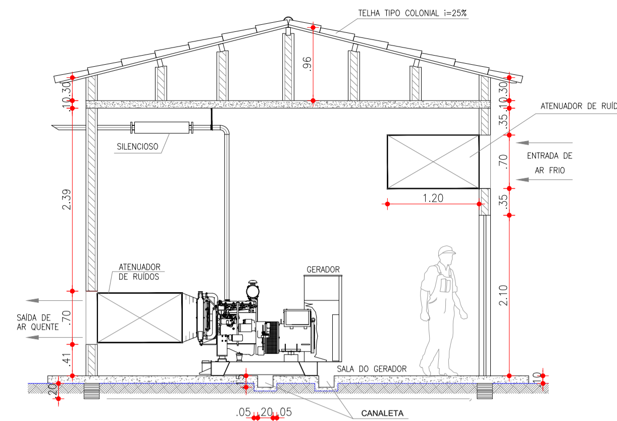
5 CORTE C-C ESCALA: 1/50
