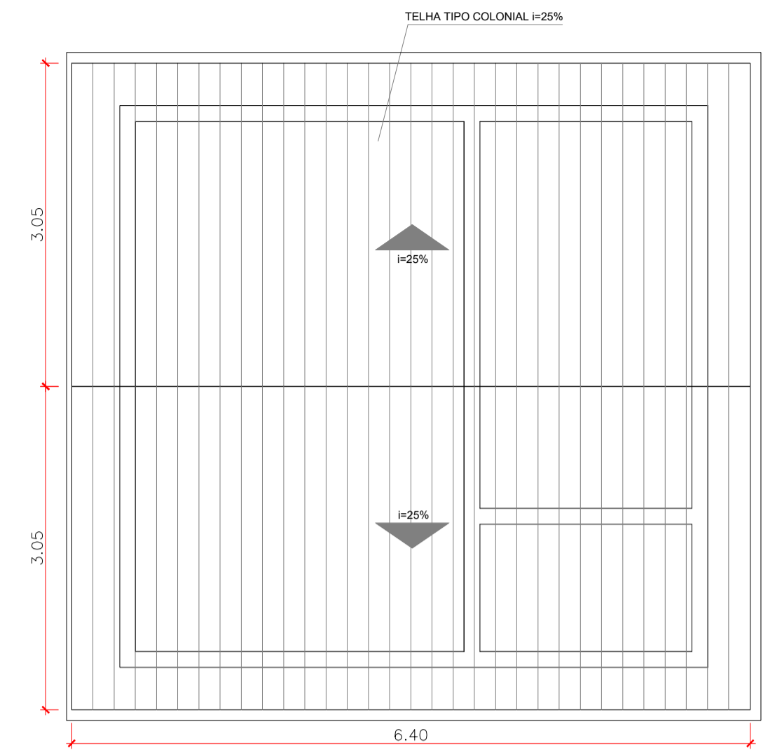
2 PLANTA DE COBERTA ESCALA: 1/50
