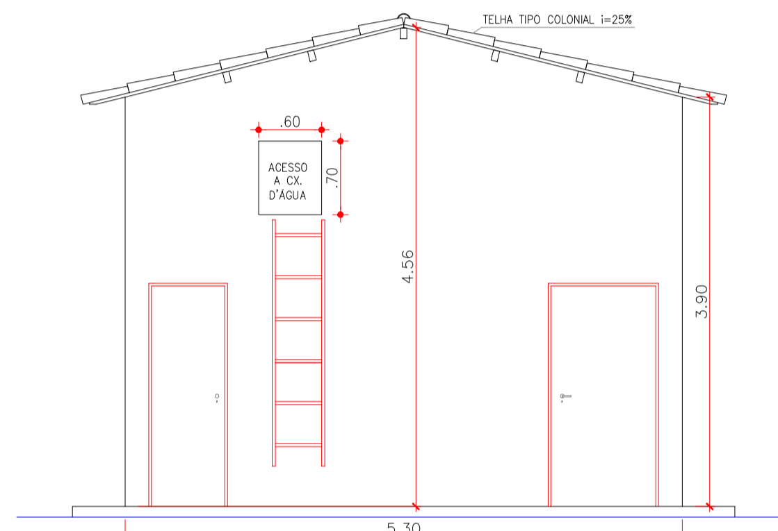
6 VISTA 01 ESCALA: 1/50
