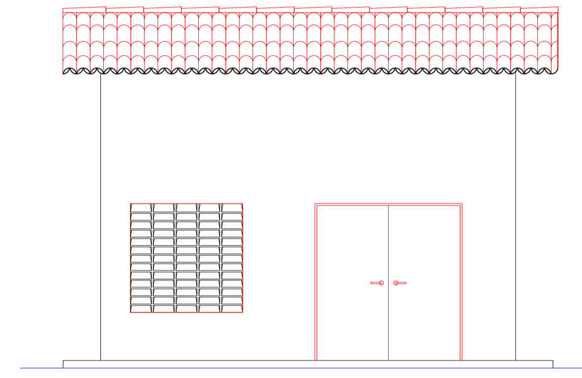
7 VISTA 02 ESCALA: 1/50
