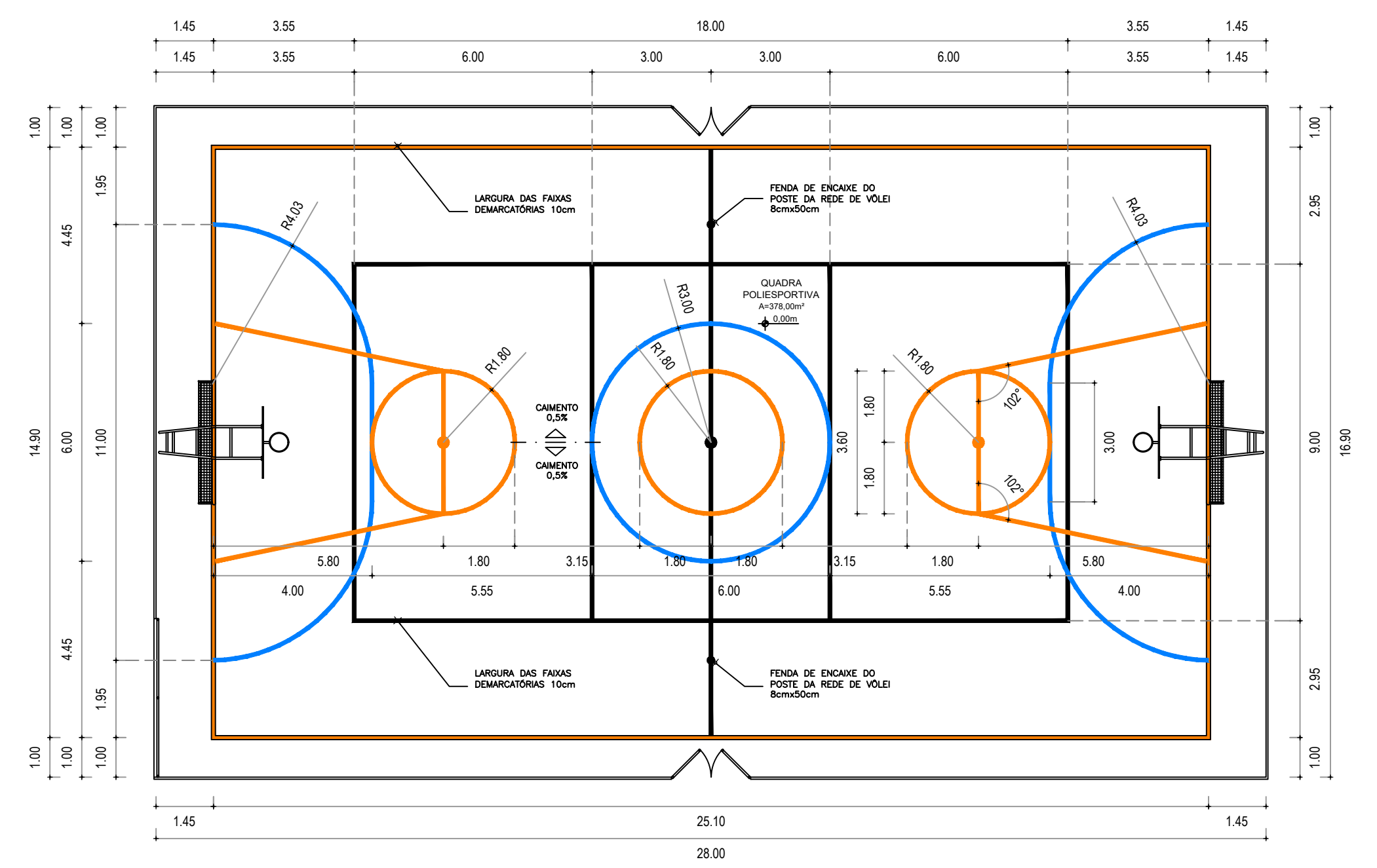
2 MEDIDAS DEMARCAÇÃO QUADRA ESCALA 1/75
