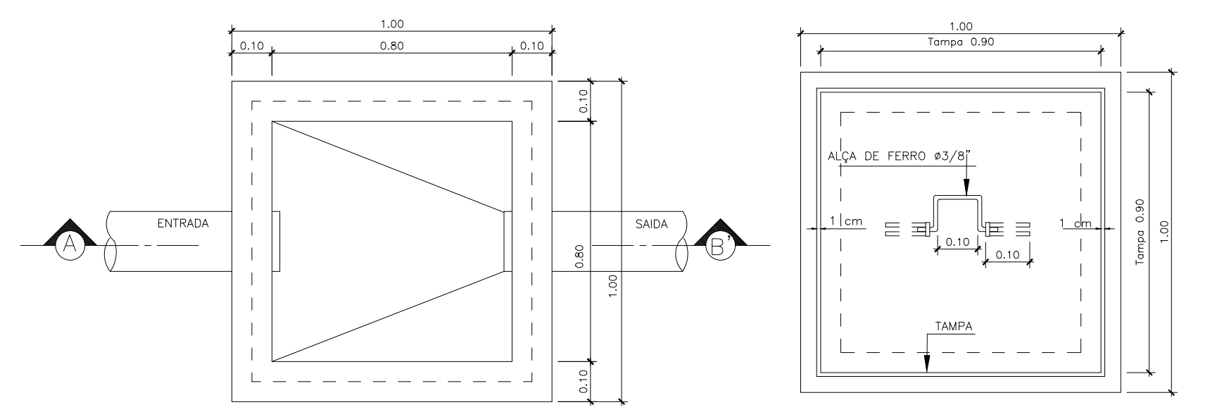
PLANTA BAIXA
