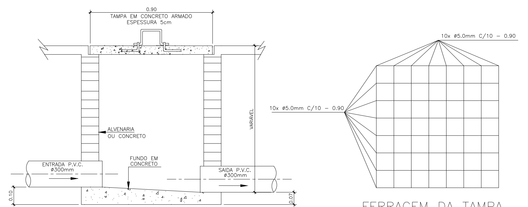
CORTE - A B'
