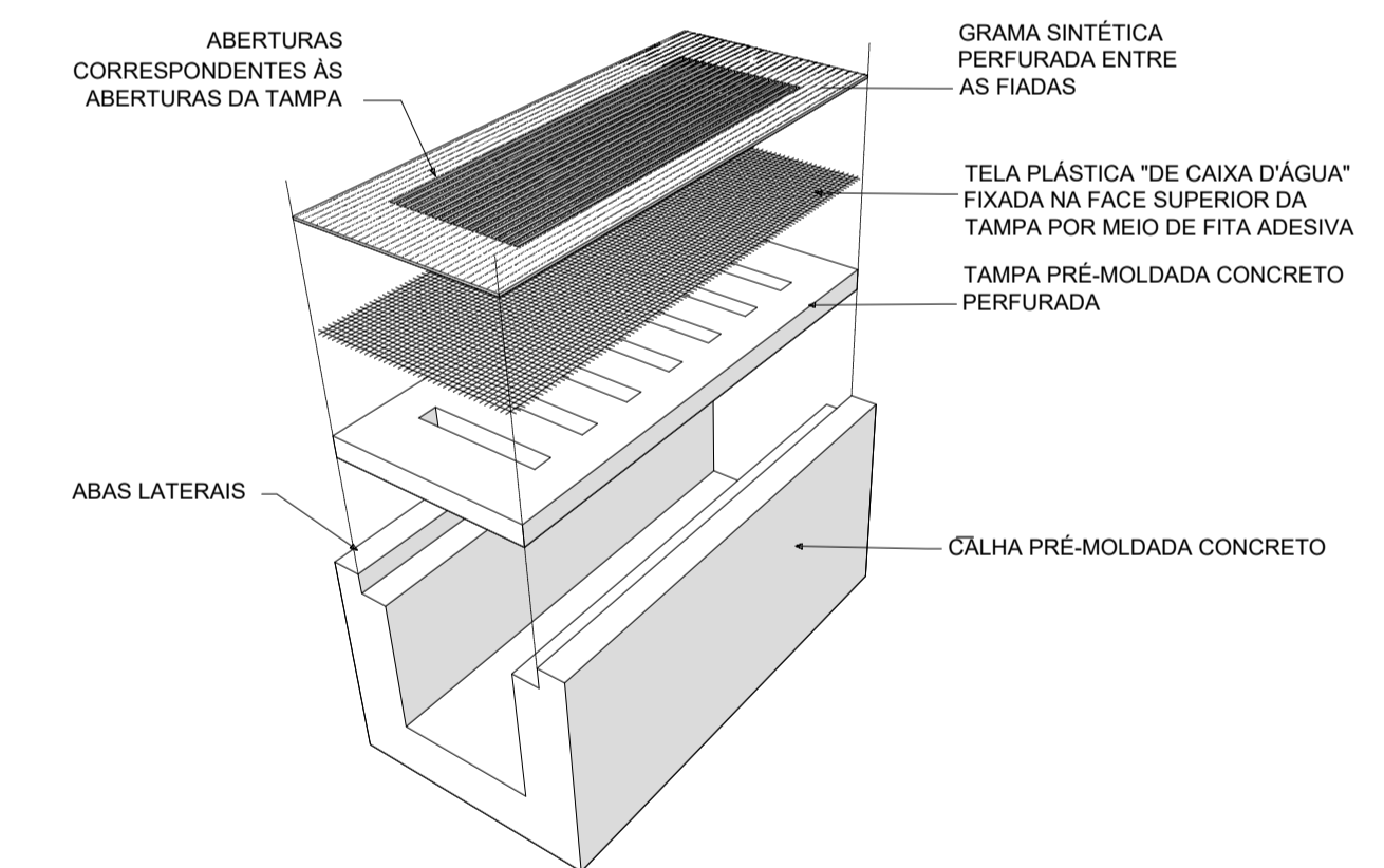
DETALHE CALHA DE DRENAGEM
