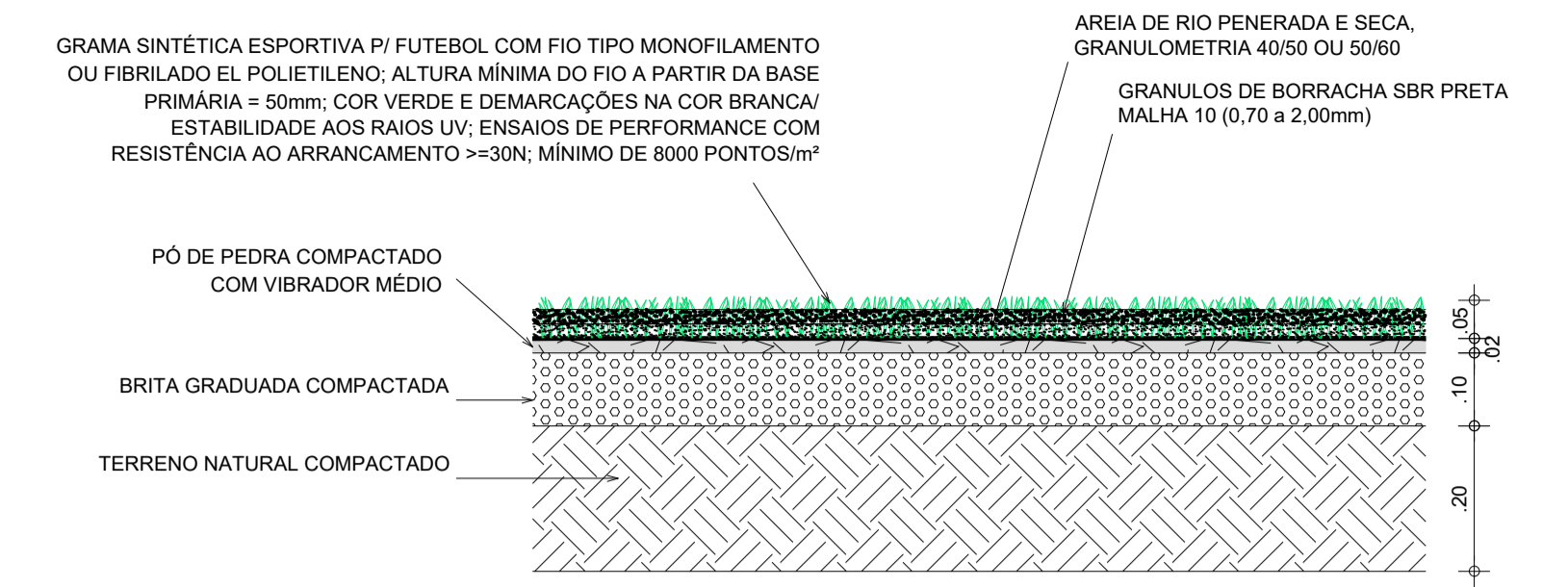
DETALHE DISPOSIÇÃO GRAMADO SINTÉTICO
