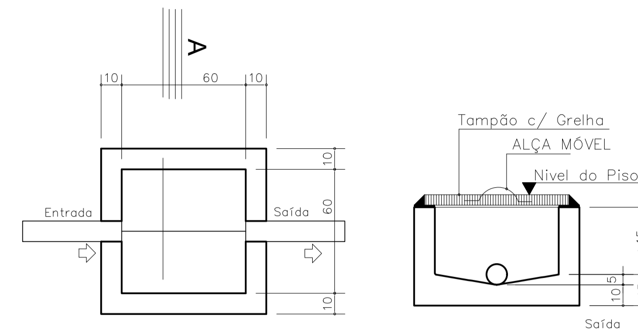
PLANTA CORTE AA CAIXA DE CAPTAÇÃO DE ÁGUAS PLUVIAIS - ESC. 1:20
