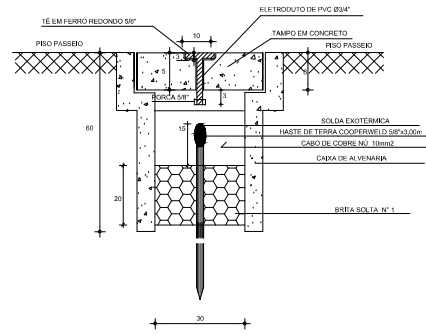
DETALHE ATERRAMENTO SEV ESCALA
