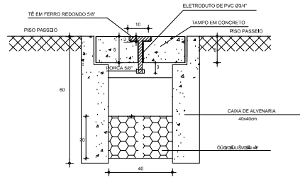
DETALHE CX. DE PASS. SEV ESCALA
