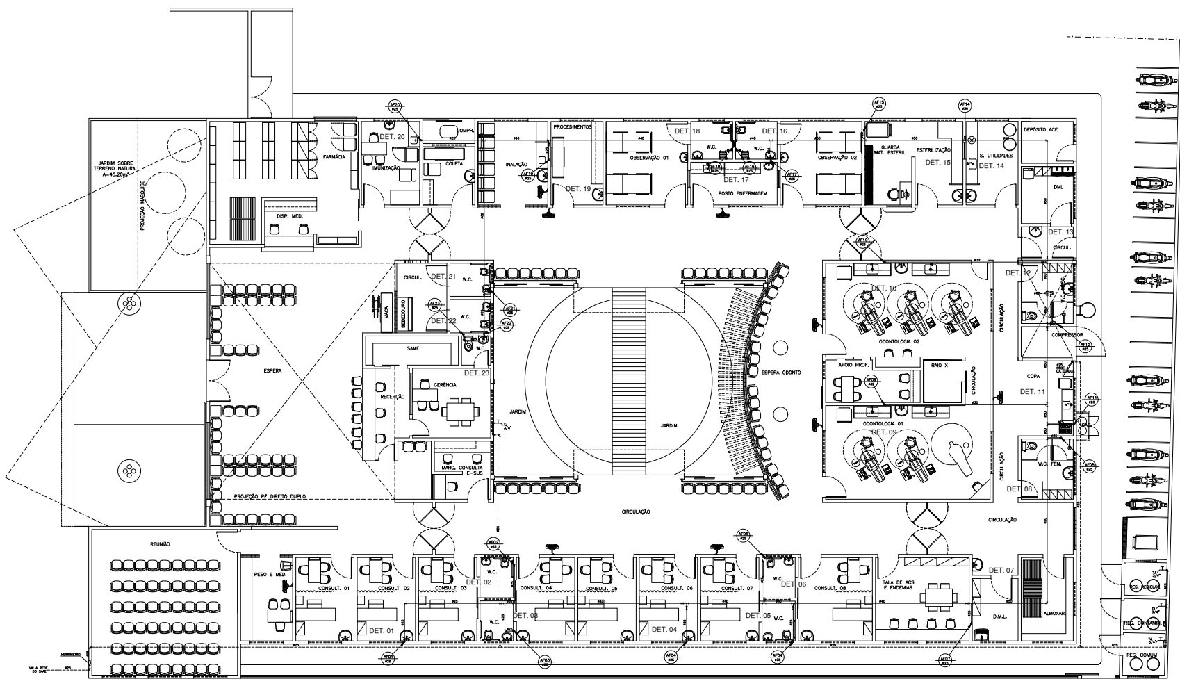
PLANTA BAIXA ESCALA 1/75
