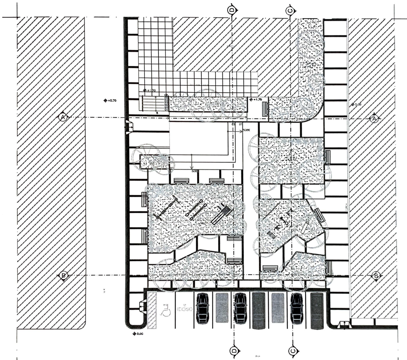
01 PLANTA BAIXA 1/100
