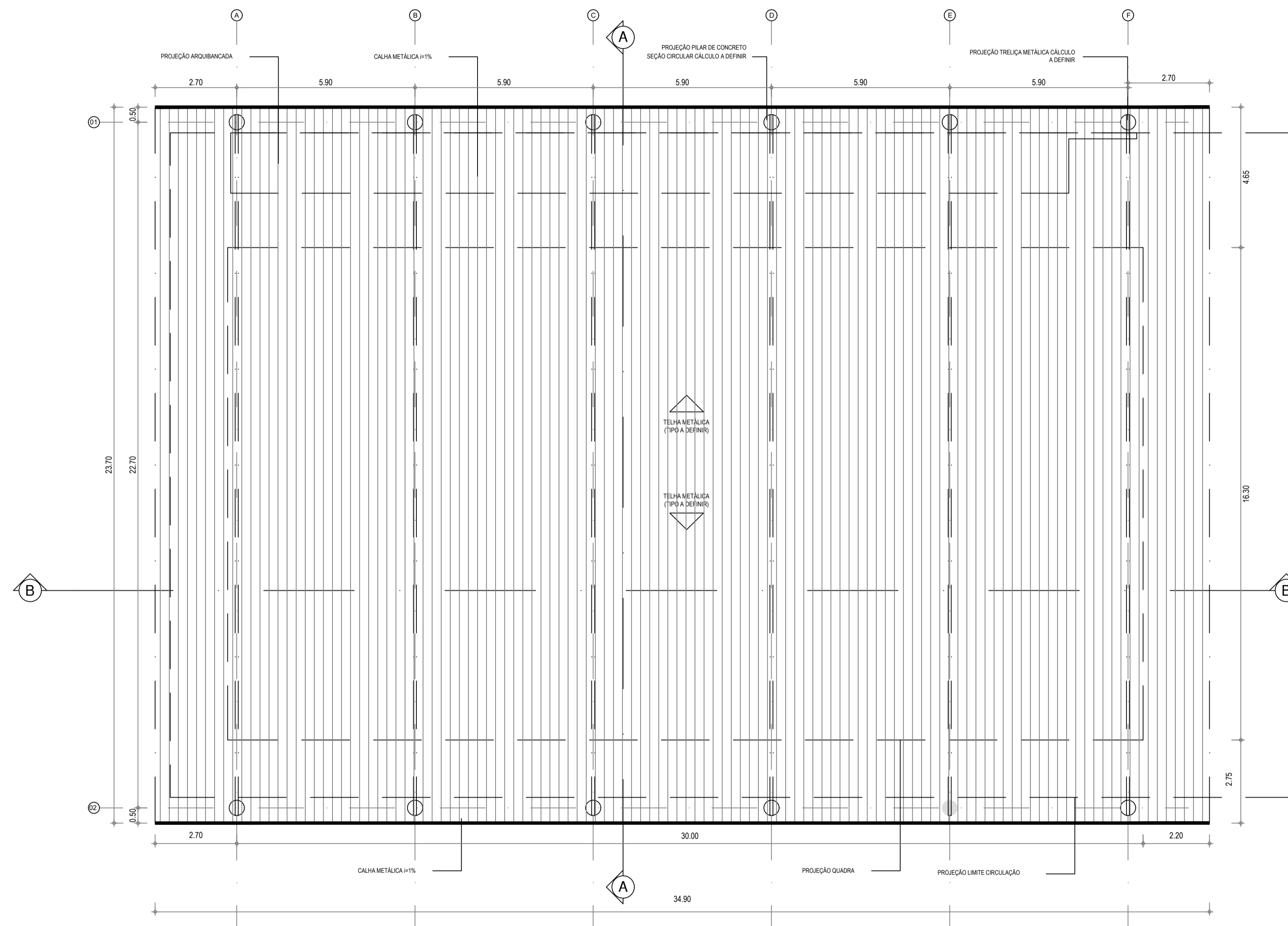
1 PLANTA DE COBERTA ESCALA 1/100
