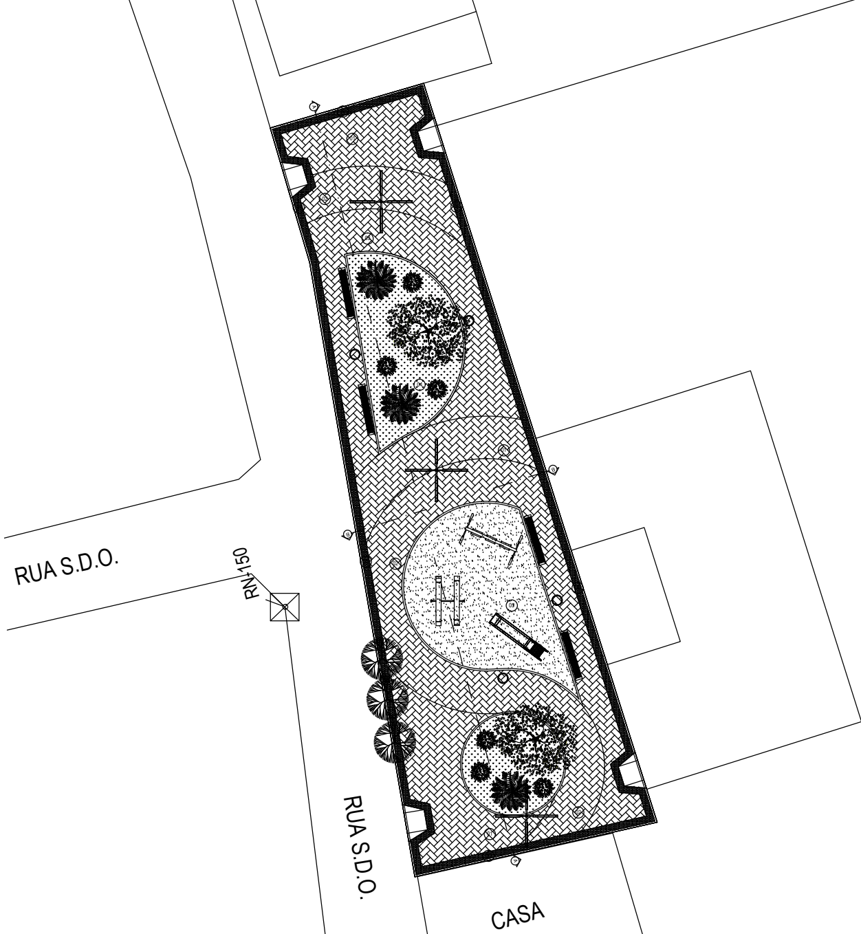
1 PLANTA BAIXA GERAL ESCALA: 1:100
