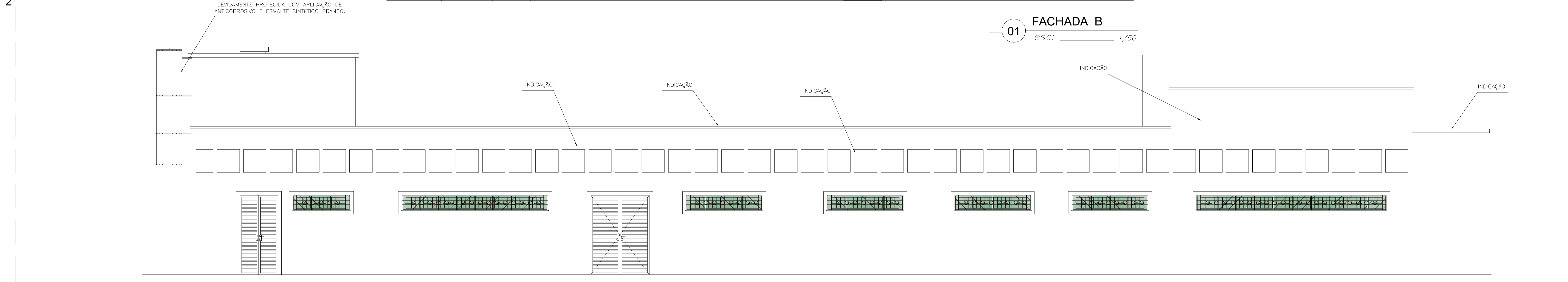
02 FACHADA C esc: 1/50
